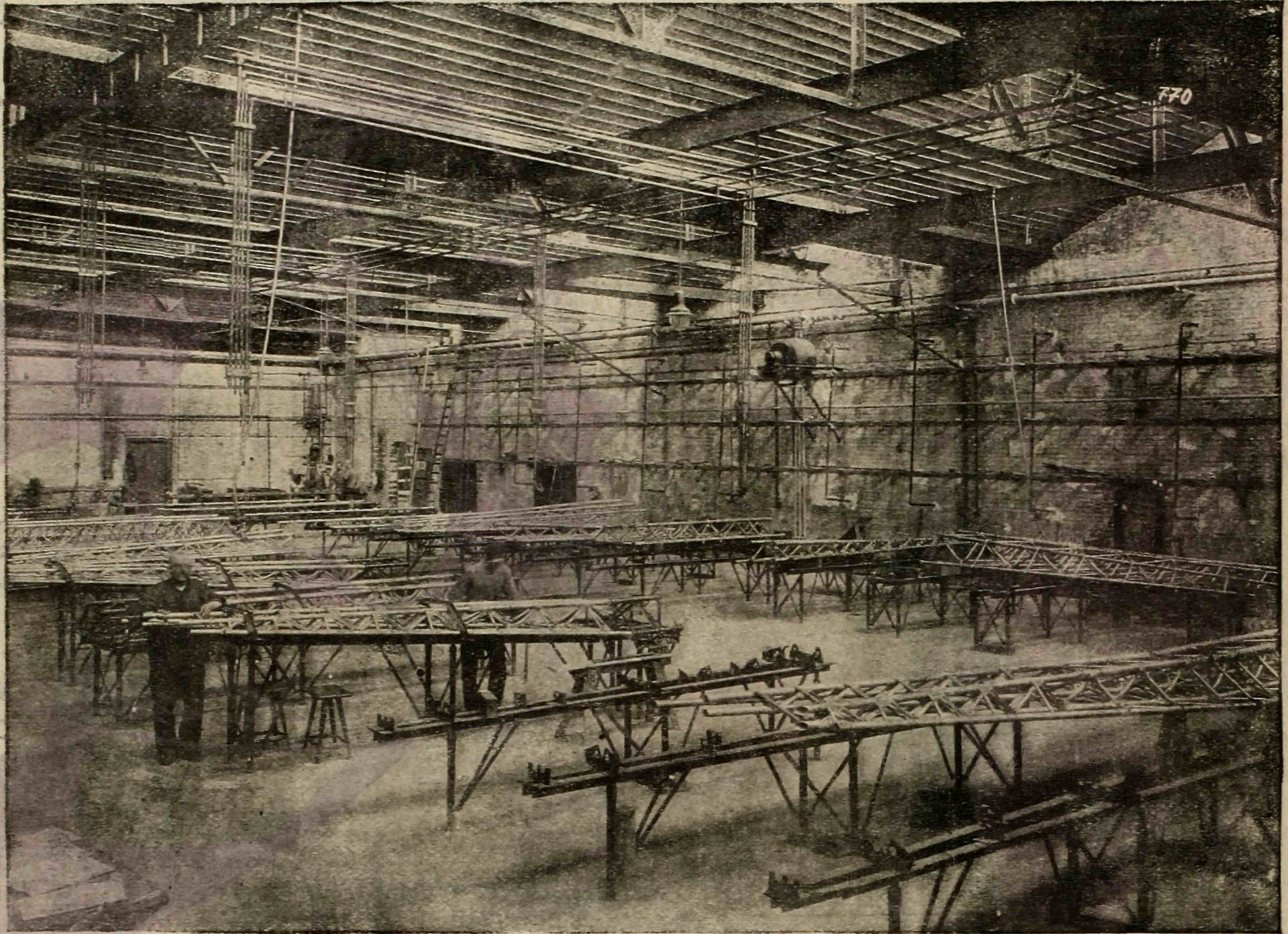
Рис. 1. Вид мастерской, где из отдельных дураллюминиевых трубок составляются продольные крепления крыльев Юнкера (лонжероны).
