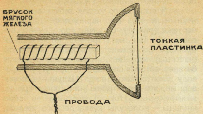
Рис. 3. Простая схема телефонного аппарата.
