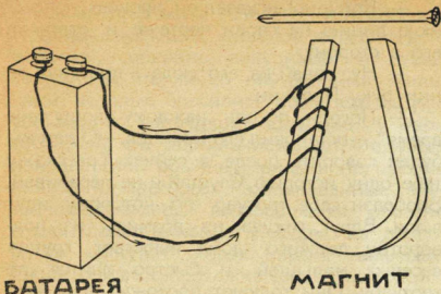
Рис. 2. Как гвоздь вызывает в проводе электрический ток.
