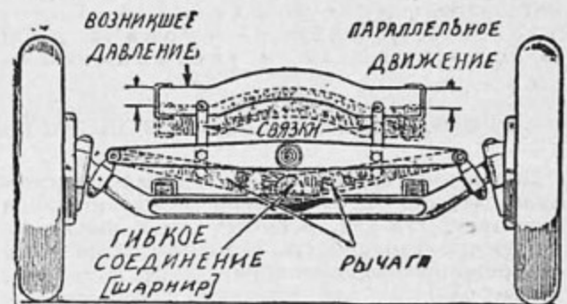
Схема устройства нового стабилизатора.
