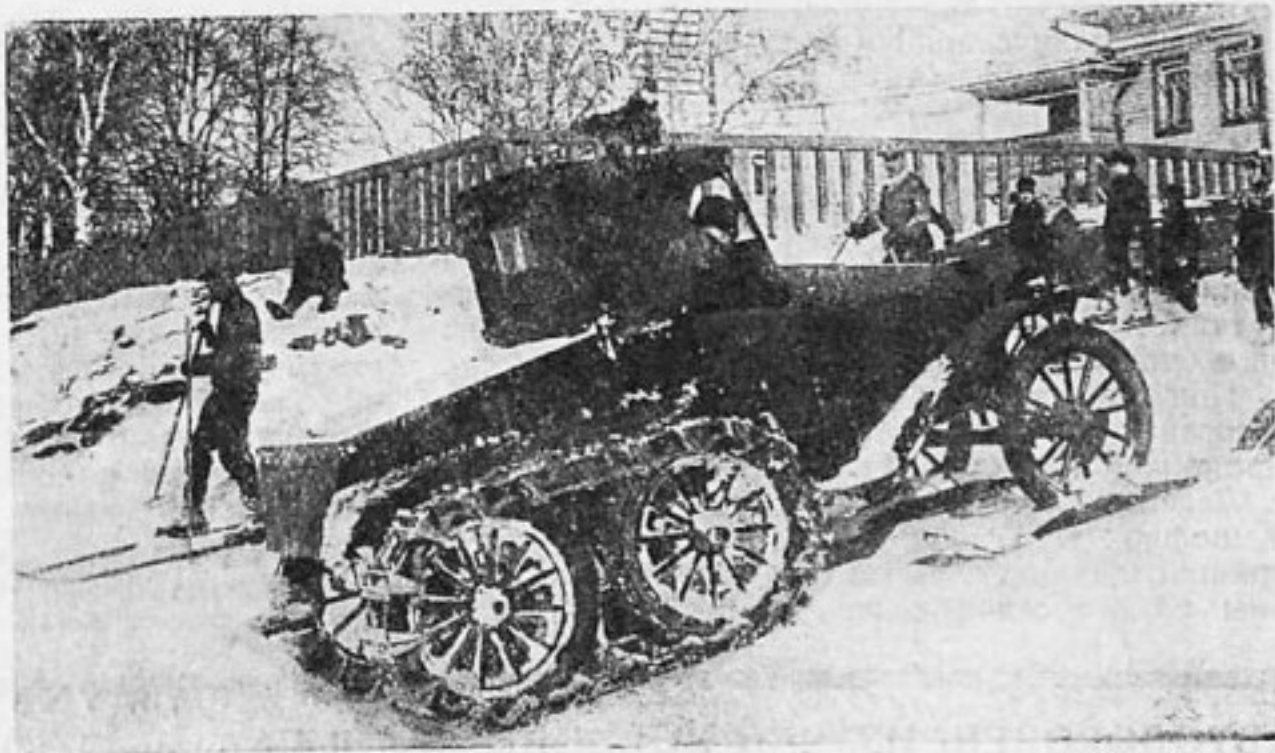
Гусеничные автосани на подъеме
