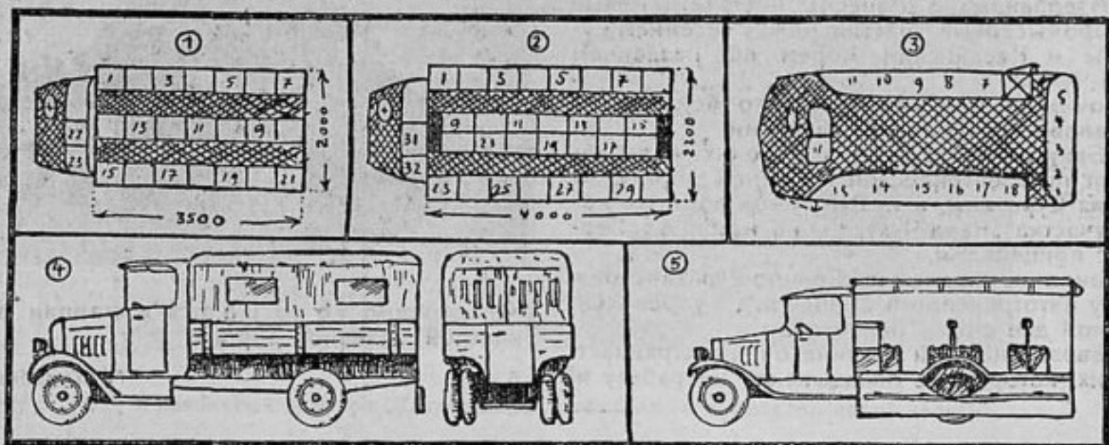
1. Устройство сидений в 2 1 / 2 -тонном рабочем автобусе. 2. То же в 5-тонном. 3. Рабочий автобус Геншеля. 4. Комбинированный автобус МАН. 5. Рабочий автобус Дюркопп.
