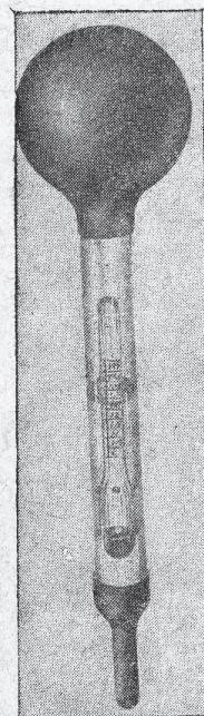
Фиг. 43. Ареометр
