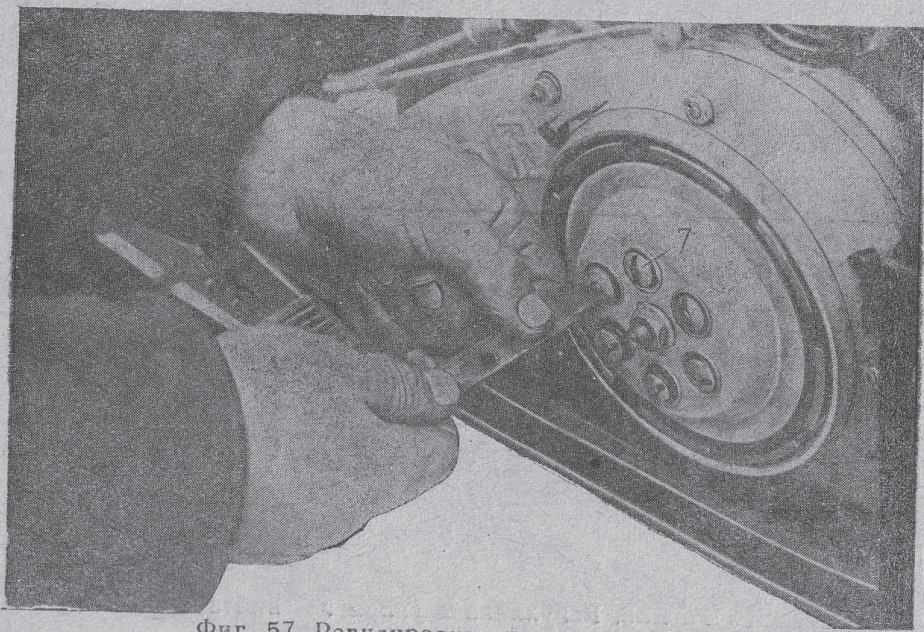
Фиг. 57. Регулировка пружин сцепления
