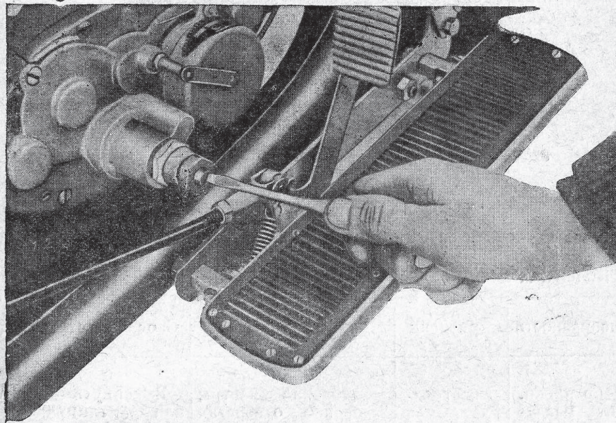
Фиг. 21. Регулирующий винт маслопровода
