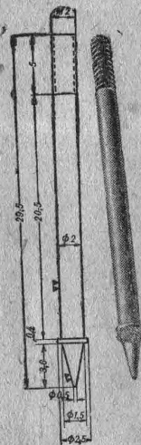
Рис. 43. Сердечник свечи (деталь 30).
