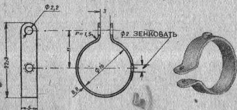
Рис. 35. Хомут прерывателя (деталь 14).
