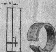
Рис. 36. Изолятор хомута (деталь 26).
