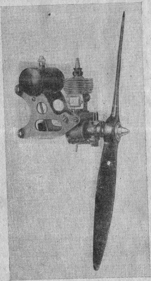
Рис. 1. Фото моторчика ПП-4.
