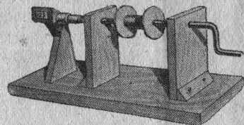
Рис. 61. Станочек для намотки со счетчиком.
