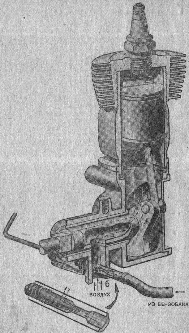
Рис. 3. Внутреннее устройство моторчика ПП-4.
