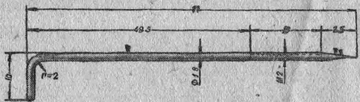
Рис. 38. Игла карбюратора (деталь 18).
