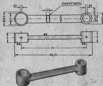
Рис. 27. Шатун (деталь 8).
