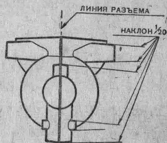
Рис. 12. Наклоны модели.
