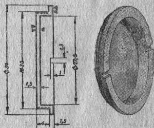
Рис. 21. Заглушка (деталь 4).
