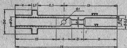
Рис. 35. Хомут прерывателя (деталь 14).
