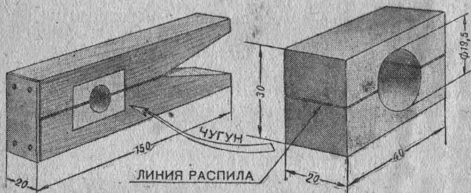
Рис. 26. Приспособление для шлифовки поршня.
