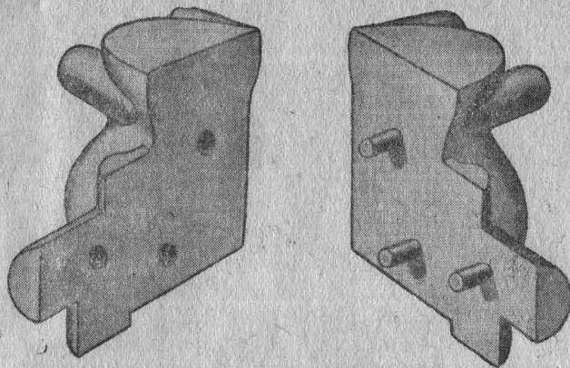
Рис. 16. Укрепление штифтов.
