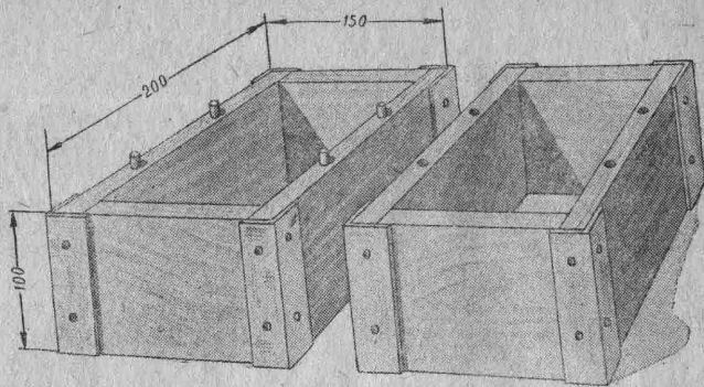
Рис. 17. Опoки.
