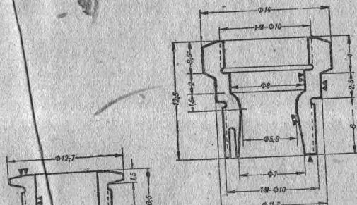
Рис. 39. Стопор иглы карбюратора (деталь 19).
