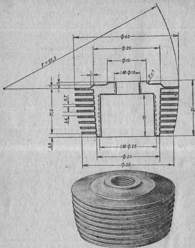
Рис. 23. Головка цилиндра (деталь 2).
