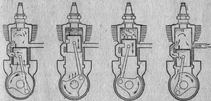
Рис. 6, 7, 8 и 9. Схемы работы двигателя.
