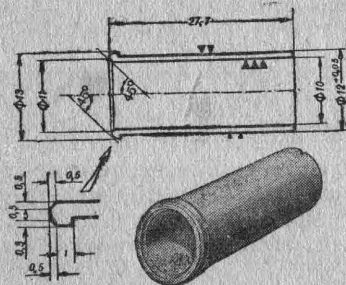
Рис. 20. Втулка вала (деталь 5).
