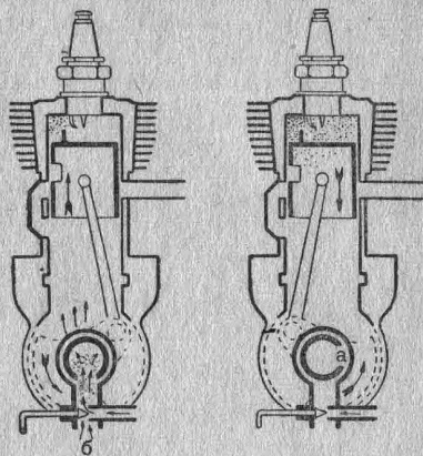
Рис. 4 и 5. Газораспределение.
