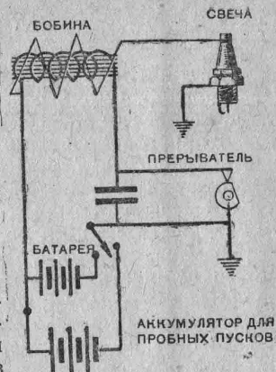
Рис. 58. Схема зажигания.
