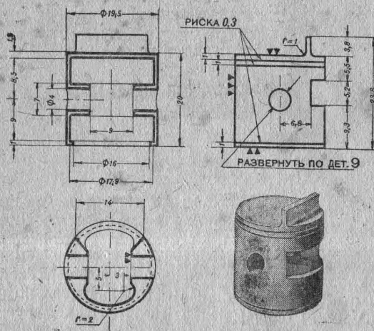
Рис. 25. Поршень (деталь 7).
