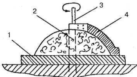
Рис. 28. Основной шаблон для вазона: 1 — отмостка; 2 — первый отрезок трубы; 3 — второй отрезок трубы; 4 — шаблон
