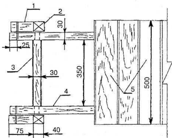
Рис. 4. Соединение ножек с рамой: 1 — проушина; 2 — ножка; 3 — поперечная рейка; 4 — продольная рейка; 5 — столешница
