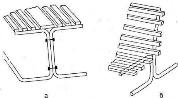
Рис. 19. Скамья с металлическим каркасом: а — без спинки;
