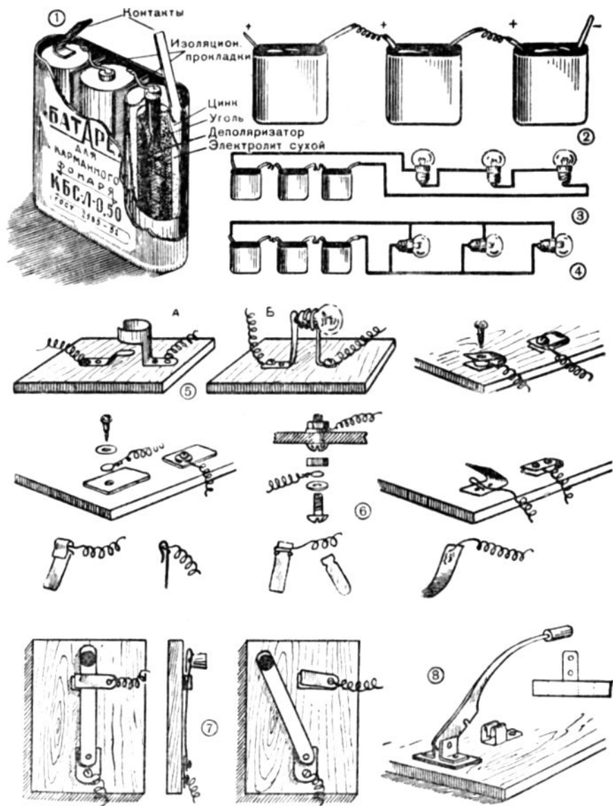
Рис. 60. Использование батареек для карманного фонаря:
