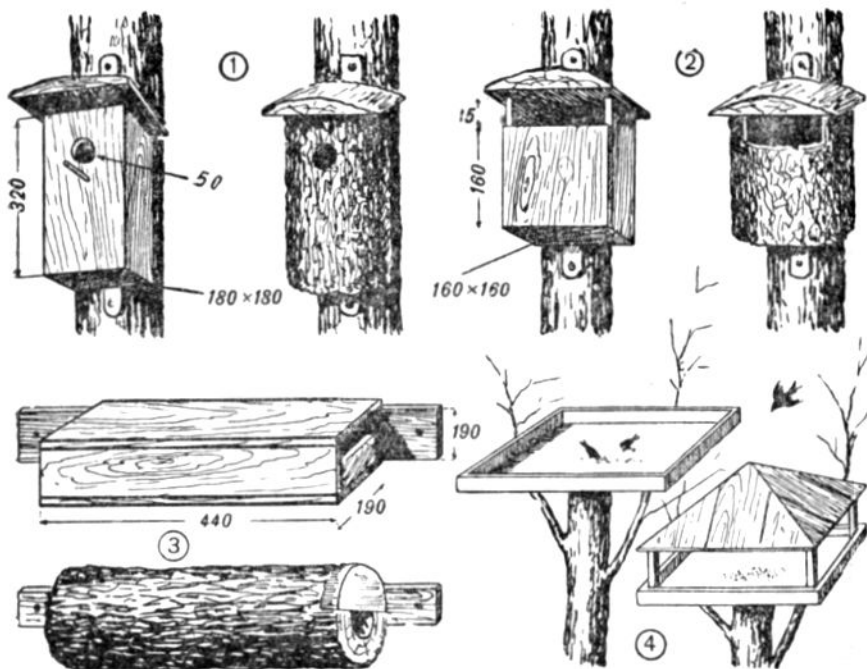
Рис. 116. Птичьи домики и кормушки:
