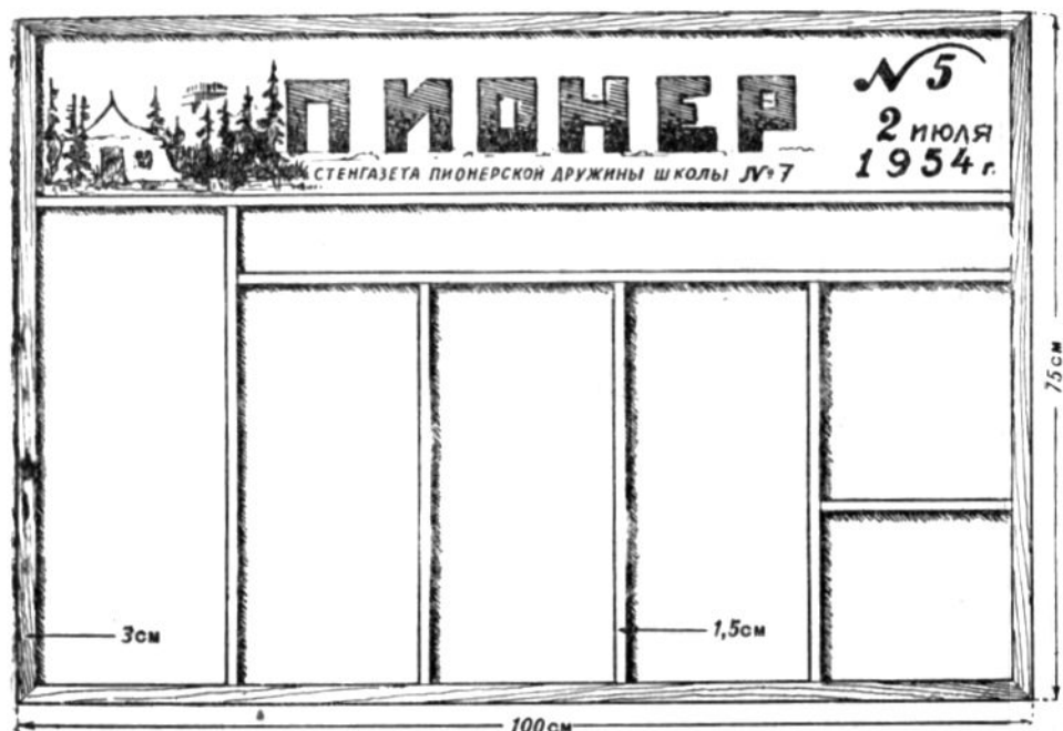
Рис. 95. Щит для стенной газеты
