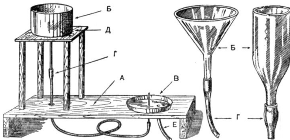
Рис. 73. Модель фонтана.
