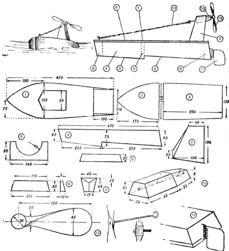
Рис. 138. Модель глссера с резиновым мотором:
