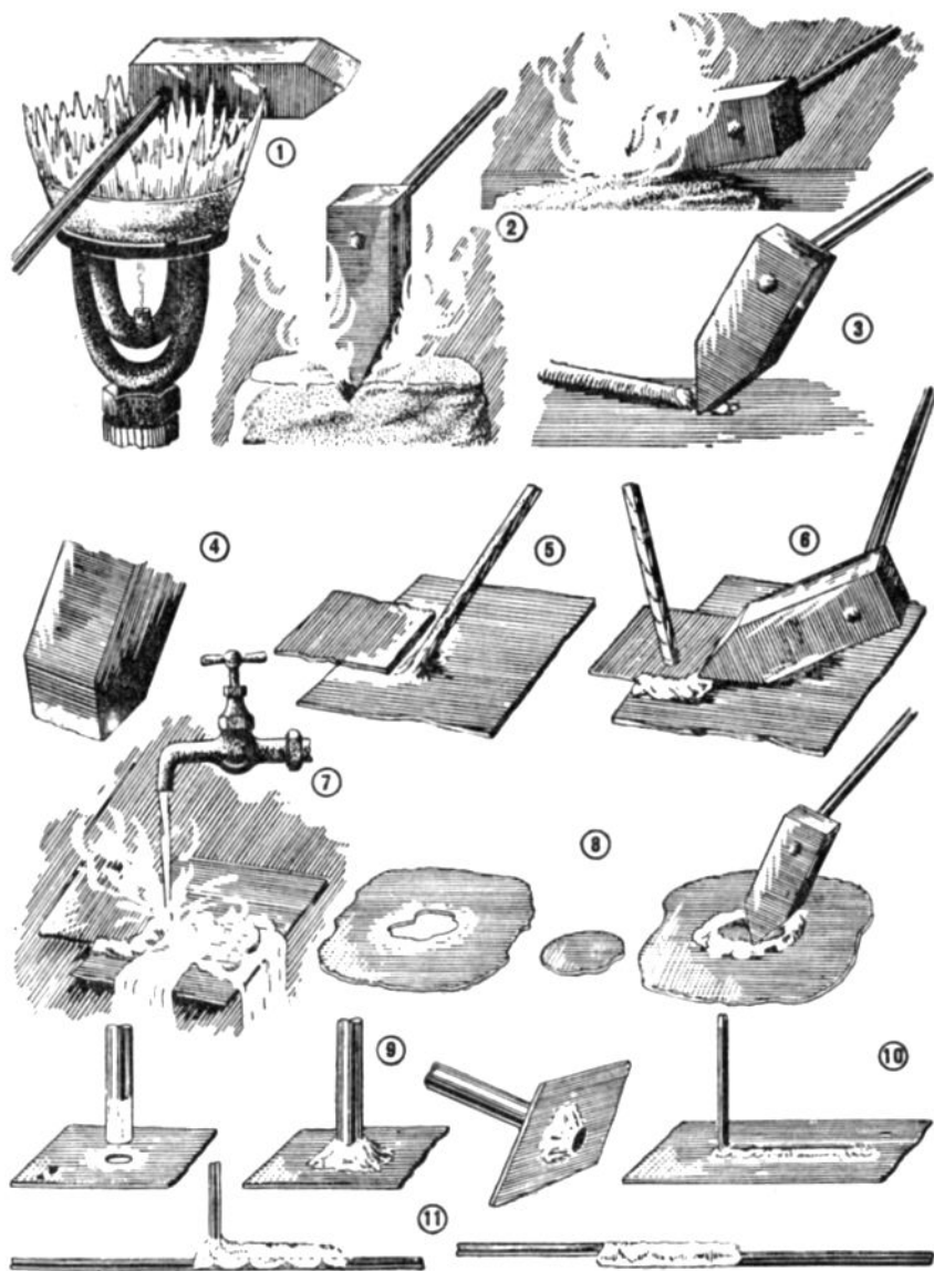
Рис. 56. Как паять:
