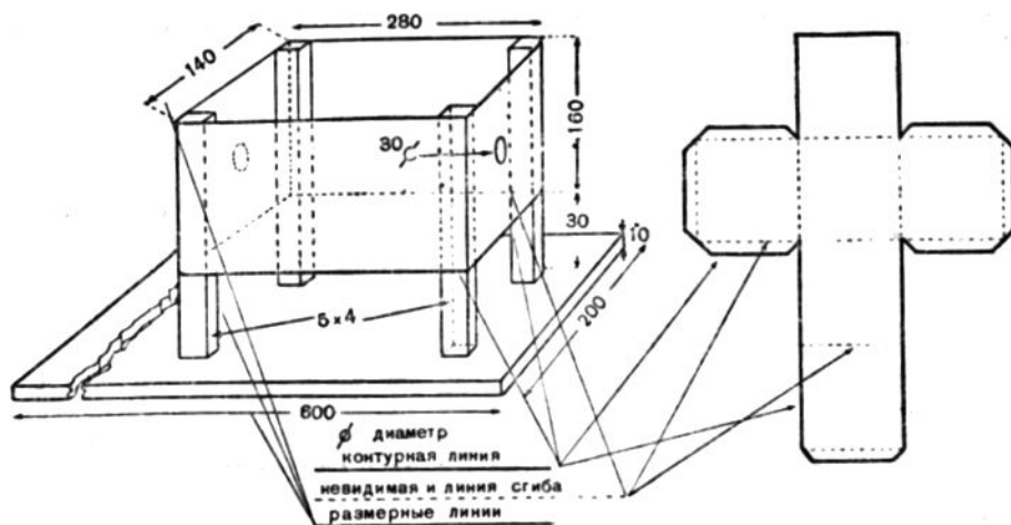
Рис. 61. Обозначения на чертежах и эскизах.
