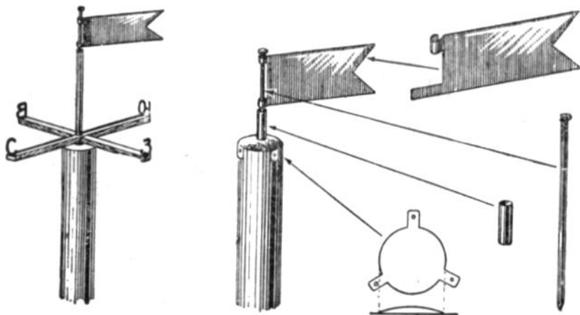
Рис. 78. Простейший флюгер.
