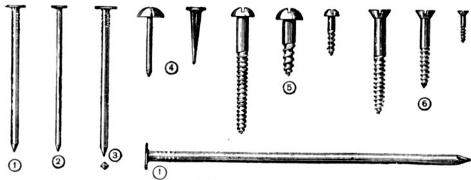
Рис. 30. Гвозди и шурупы:
