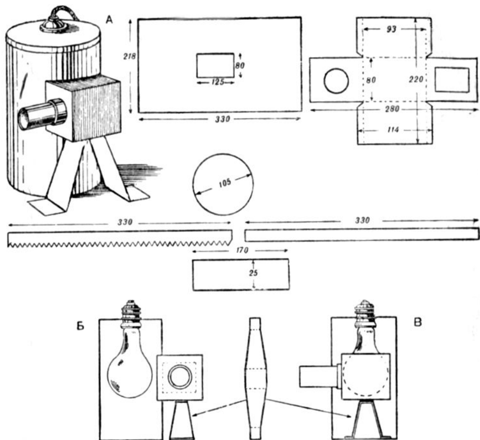
Рис. 103. Простейший эпидиаскоп:
