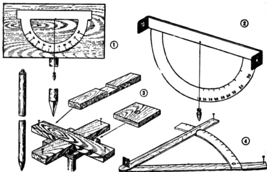
Рис. 79. Угломеры:
