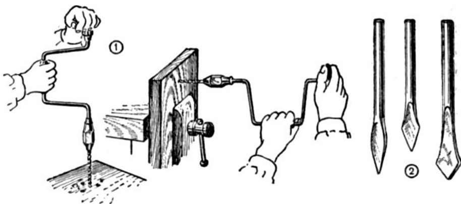
Рис. 29. Как сверлить отверстия:
