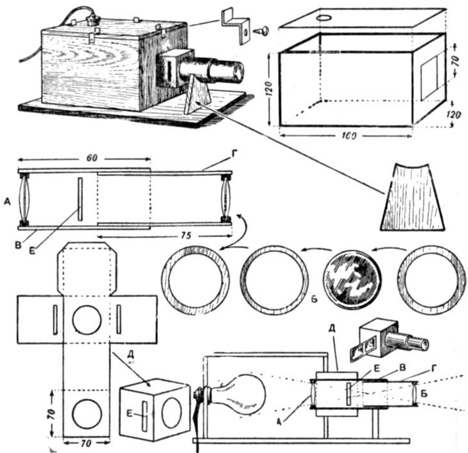
Рис. 102. Проекционный фонарь для диапозитивов:
