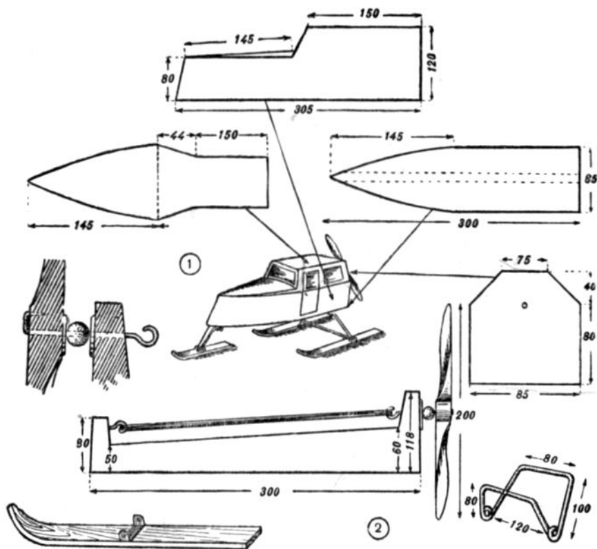
Рис. 151. Модель аэросаней с резиновым мотором: 1 — общий вид саней; 2 — резиномотор и винт.
