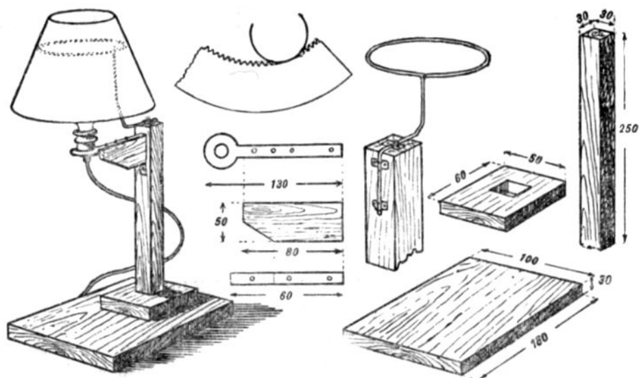
Рис. 130. Настольная лампа.
