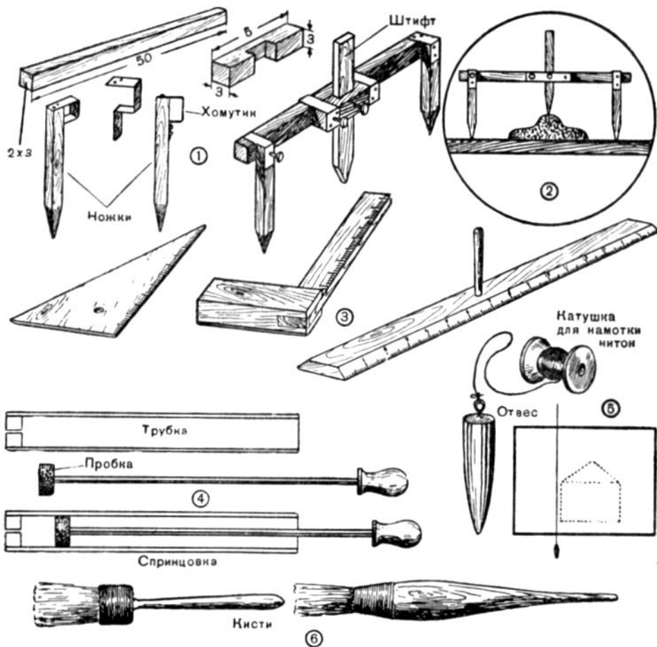
Рис. 256. Самодельные инструменты и приспособления, необходимые при лепке: 1 — мерник и его изготовление; 2 — измерение мерником высоты модели; 3 — угольники и линейка; 4 — спринцовка и ее детали; 5 — отвес и образование им линии; 6 — кисти.
