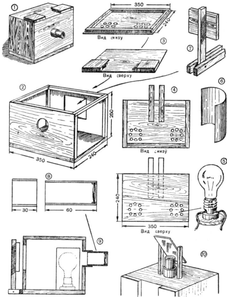
Рис. 104. Эпидиаскоп с двумя лампами:
