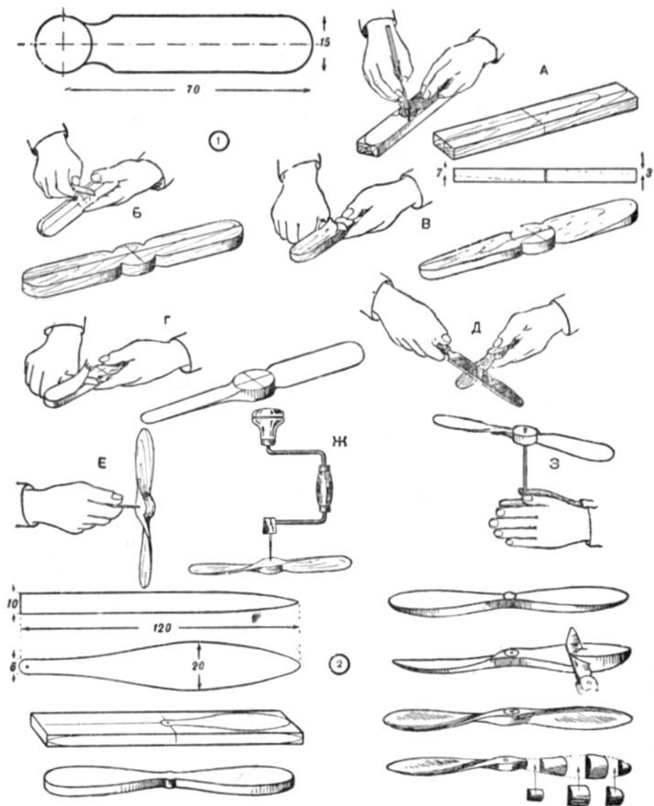
Рис. 150. Летящая модель воздушного винта (буквами указана последовательность работы):
