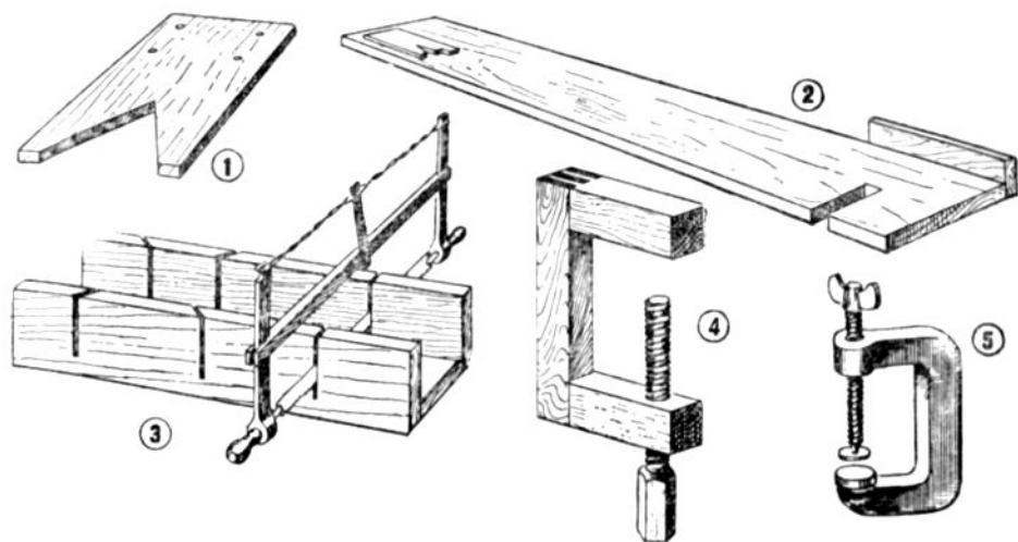
Рис. 24. Приспособления для работ по дереву:
