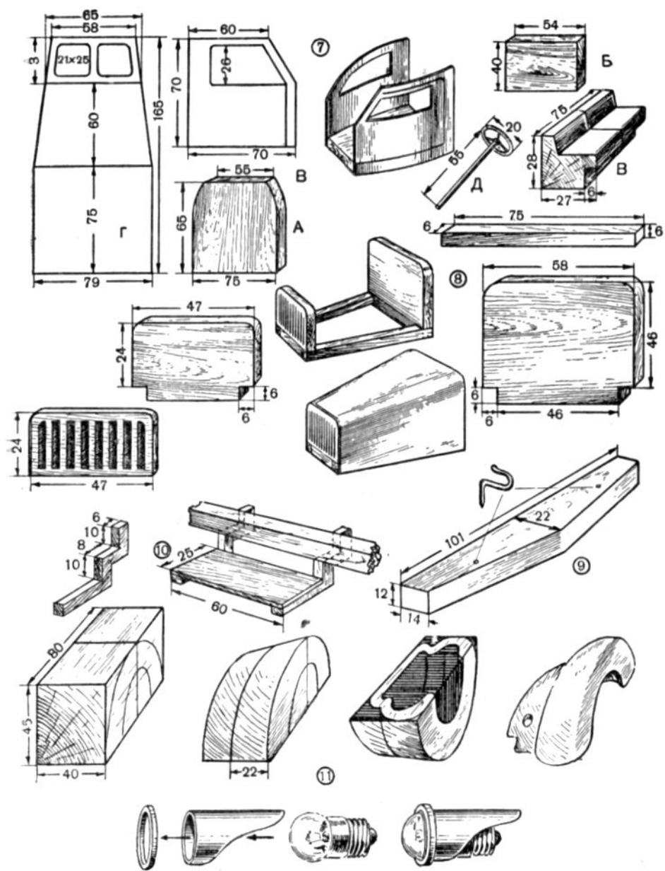
Рис. 153. Детали модели грузового автомобиля.
