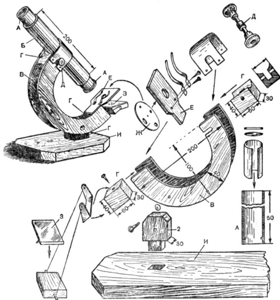
Рис. 83. Самодельный микроскоп:
