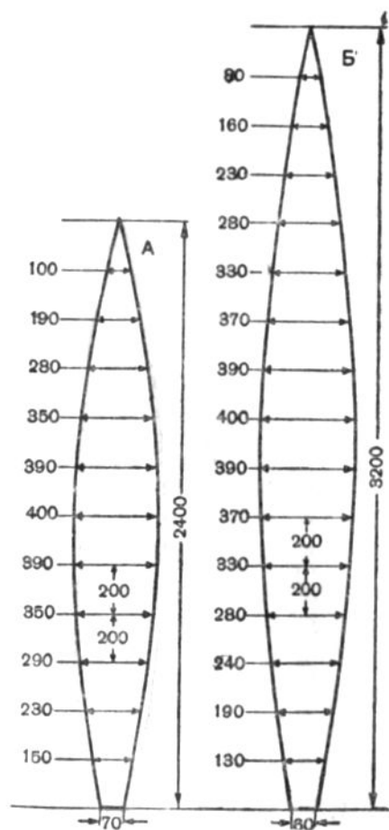
Рис. 145. Воздушный шар: разметка шаблонов полос шара: А — для шара диаметром 1,5 метра, нужно 12 полос; Б — для шара диаметром 2 метра, полос нужно 16.
