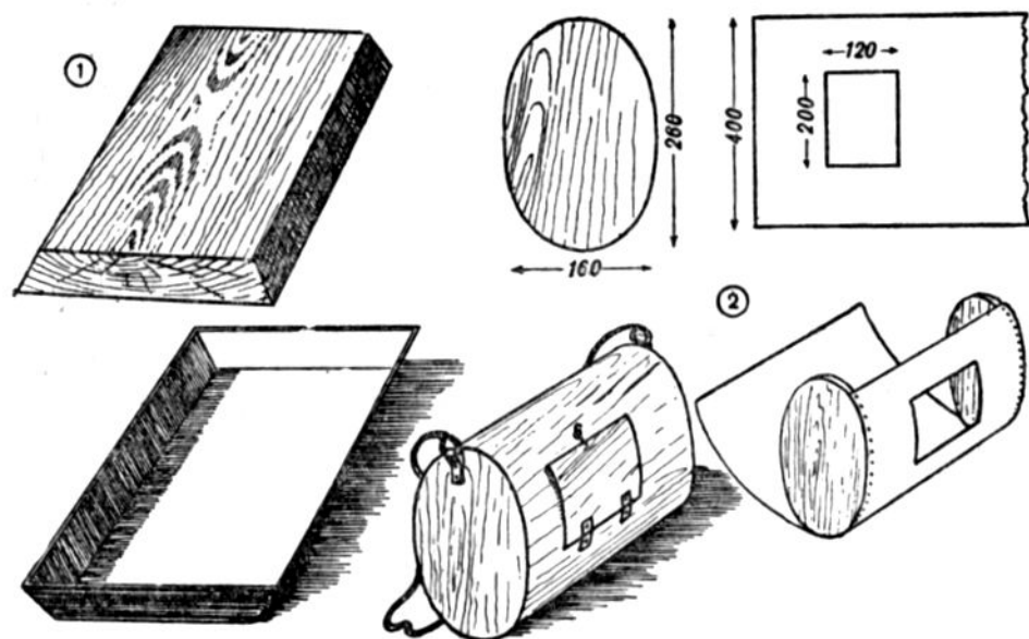
Рис. 112
