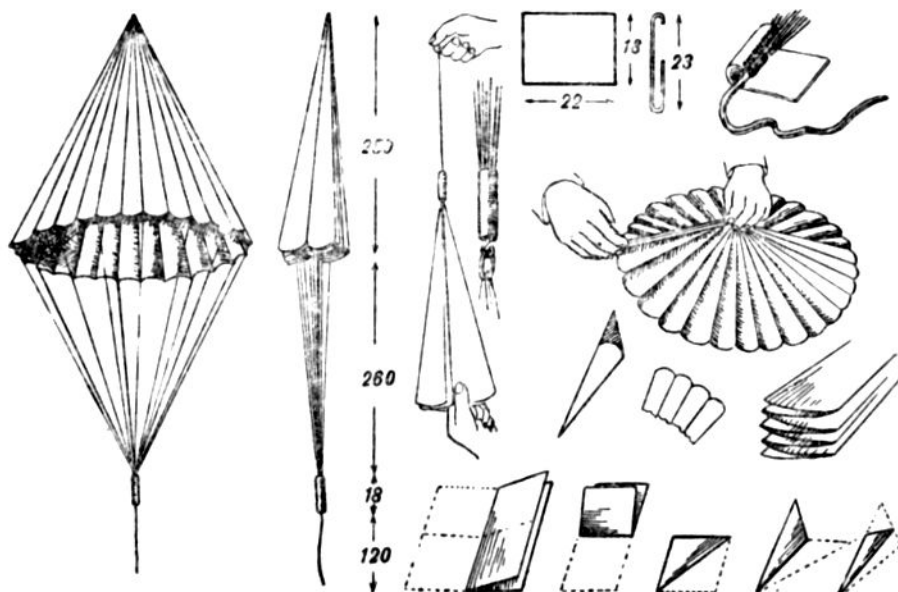
Рис. 144. Модель парашюта с самопуском.
