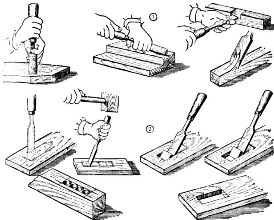
Рис. 28. Работа стамеской: 1 — разные случаи резьбы стамеской; 2 — как вырезать углубления и отверстия.
