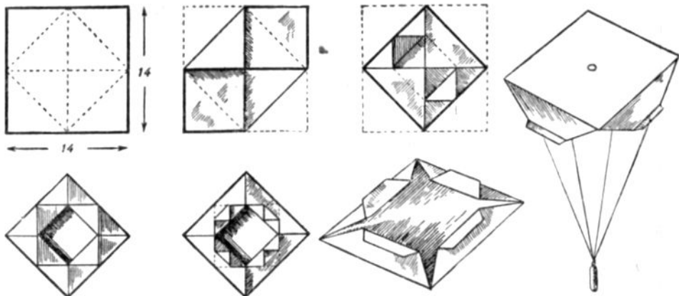
Рис. 143. Модель парашюта.
