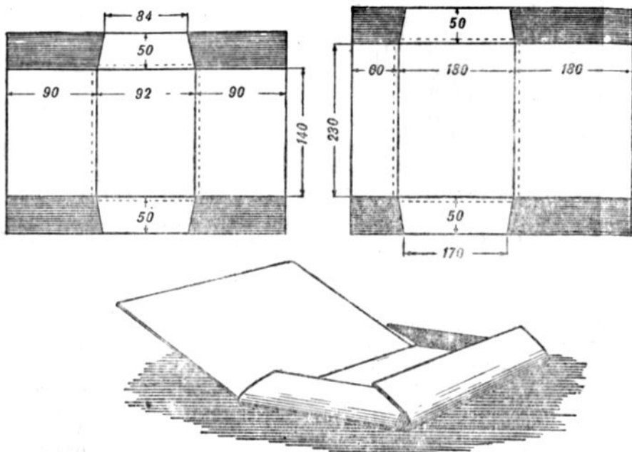
Рис. 87. Папки для фотоснимков и художественных открыток.
