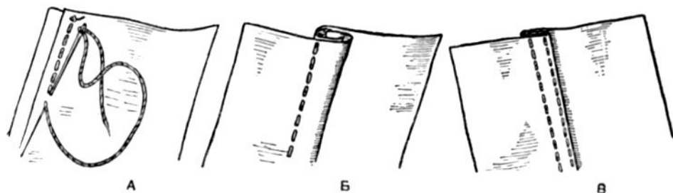
Рис. 218. Как образуется запошивочный шов (буквами указана последовательность выполнения шва).
