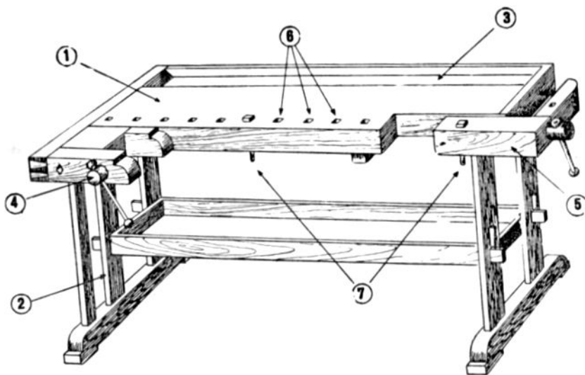
Рис. 23. Столярный верстак:
