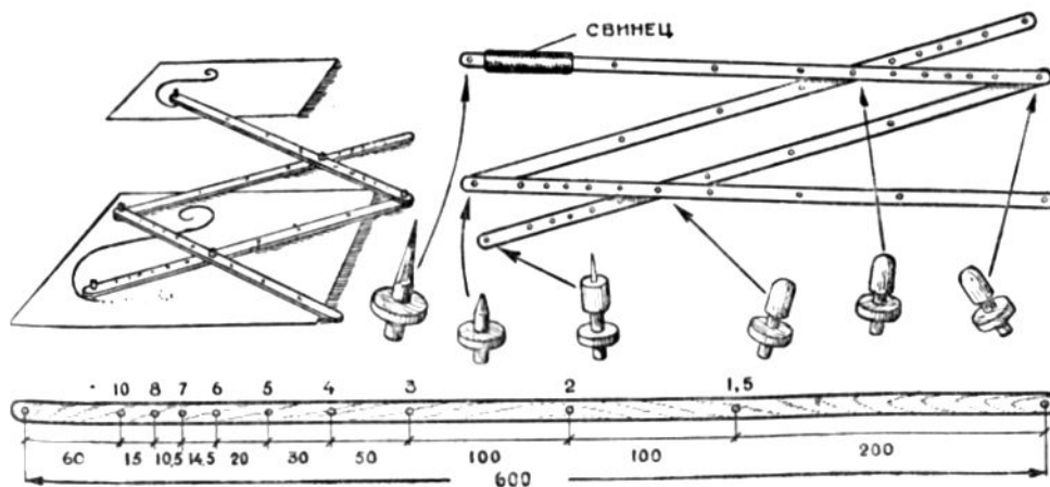
Рис. 64. Пантограф.
