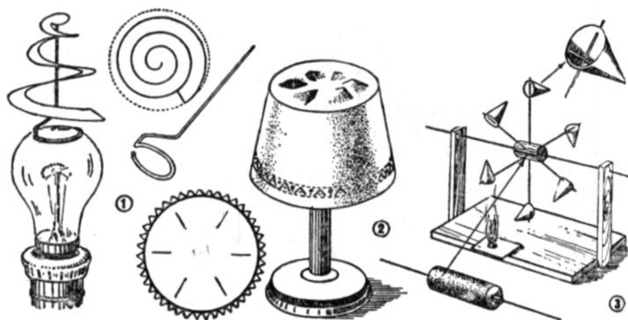
Рис. 76. Модели, демонстрирующие движение нагретого воздуха: 1 — спираль-змейка; 2 — вращающийся абажур; 3 — модель воздушного колеса.
