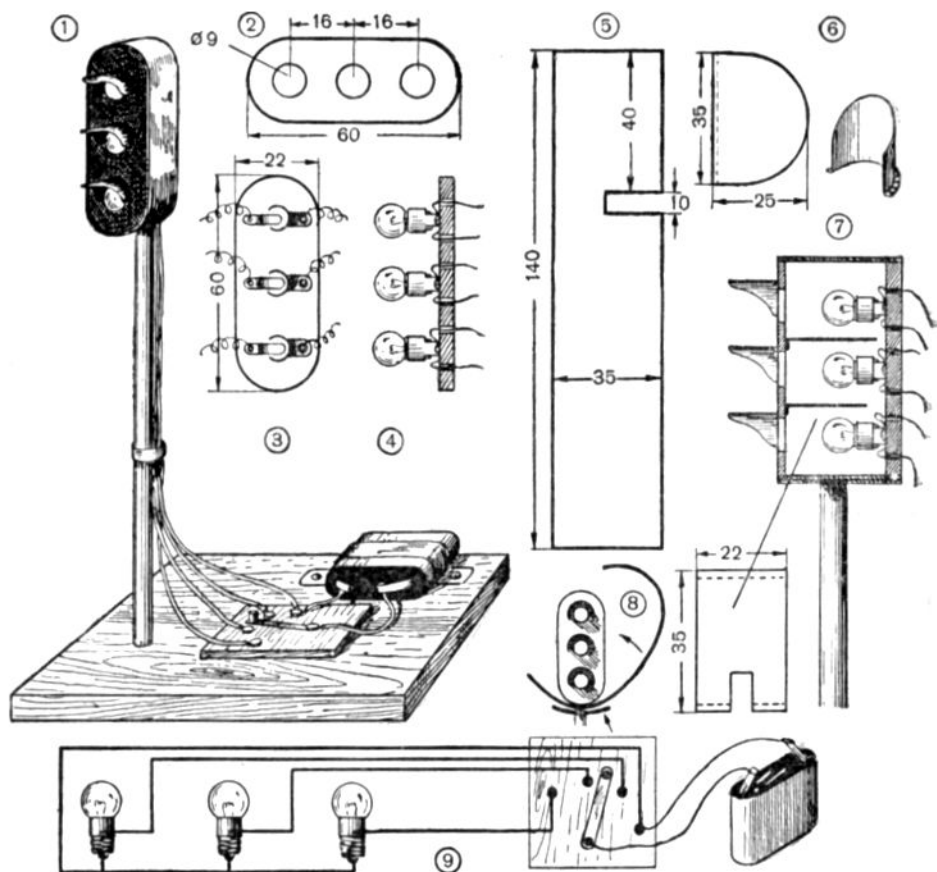
Рис. 156. Модель светофора:
