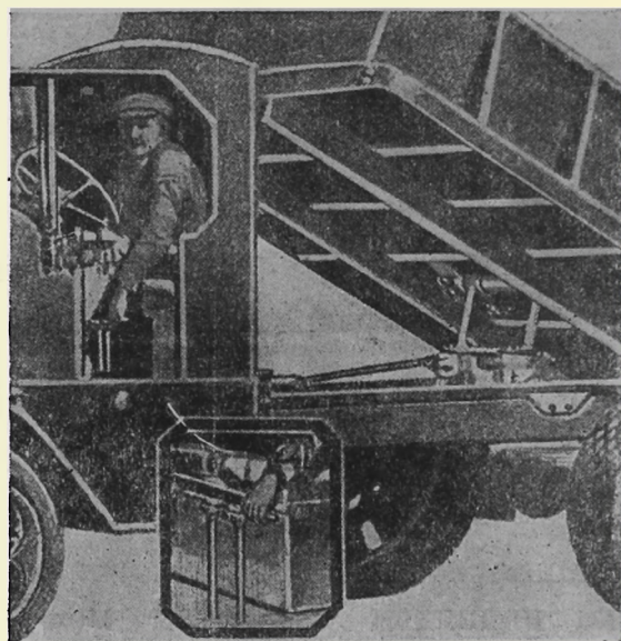
Фиг. 20. Управление гидравлическим под'емным механизмом Хилл.
