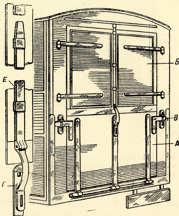
Фиг. 143. Первый тип задних двойных дверей кузова, предназначенного для перевозки различных вещей по многим адресам.
