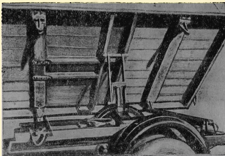
Фиг. 18. Вид кузова, поднятого механизмом Спенбург.
