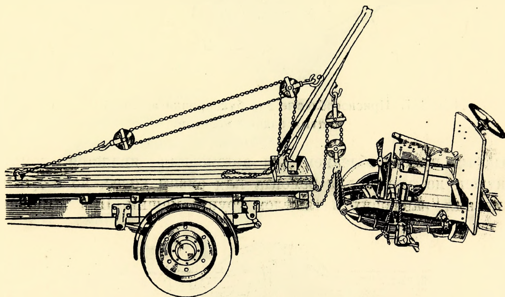
Фиг. 166. Устройство с двумя полиспастами для частичного подтягивания и буксирования попавших в аварию машин.
