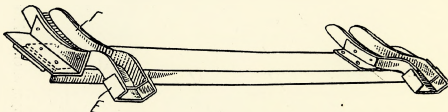
Фиг. 71. Деталь устройства опор для поддержания задних колес автомобилей в полуприцепке Мак-Гри.
