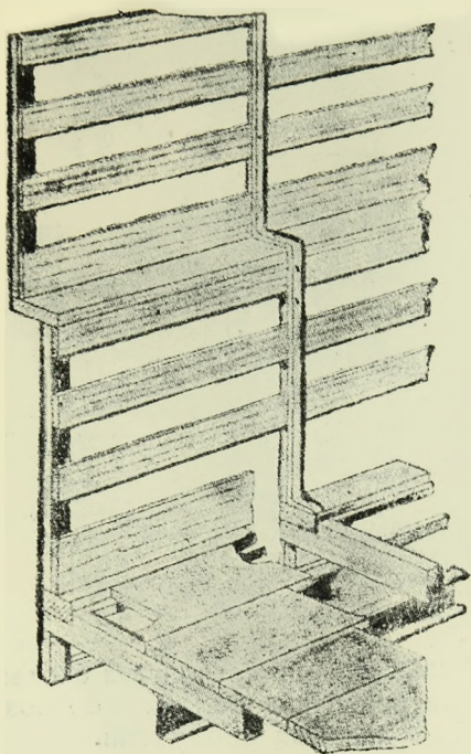
Фиг. 139. Устройство уступа в стенках кузова для наложения второго пола и двухярусной загрузки кузова.
