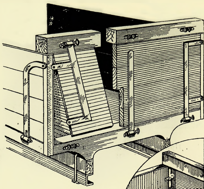
Фиг. 146. Устройство разрезного заднего борта в кузове, предназначенном для перевозки и частой разгрузки в пути материалов.
