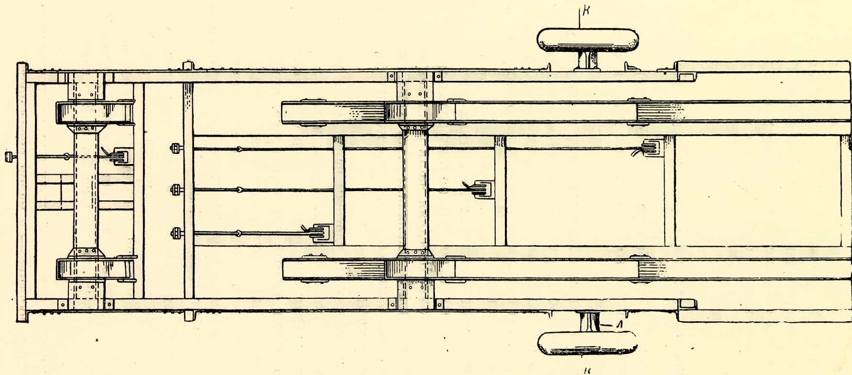
Фиг. 73. План разгруженной полуприцепки Мак-Гри.
