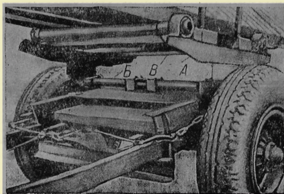
Фиг. 58. Опорная платформа полуприцепки Виккерс.
