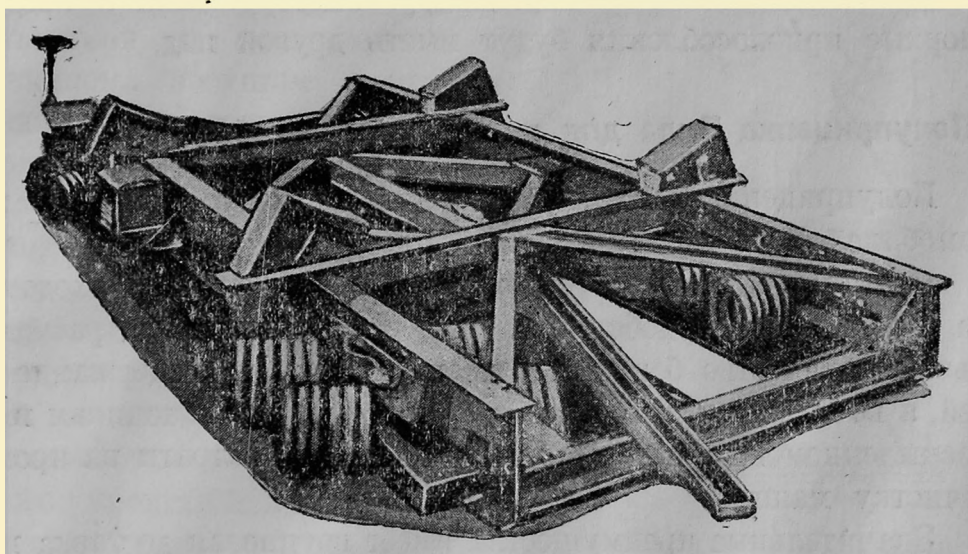
Фиг. 62. 200-тонная прицепка Лакросс.
