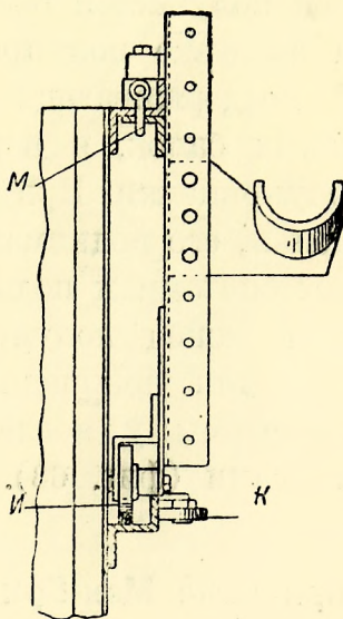
Фиг. 66. Продольное сечение одной из задних опорных тележек полуприцепки Рида.
