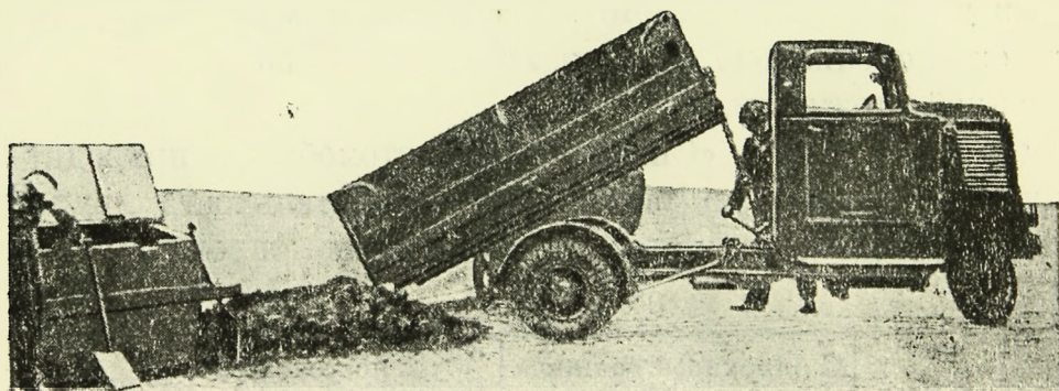
Фиг. 1. Ручной самосвал Брокгауз, приспособленный к грузовику Каррьер.
