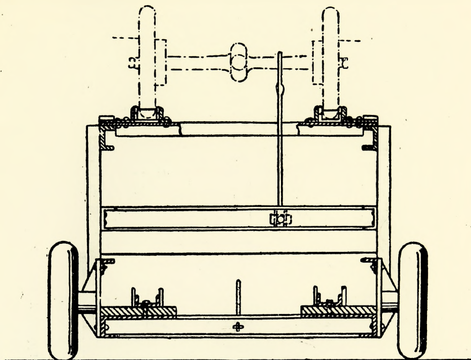
Фиг. 70. Поперечный разрез полуприцепки Мак-Гри.
