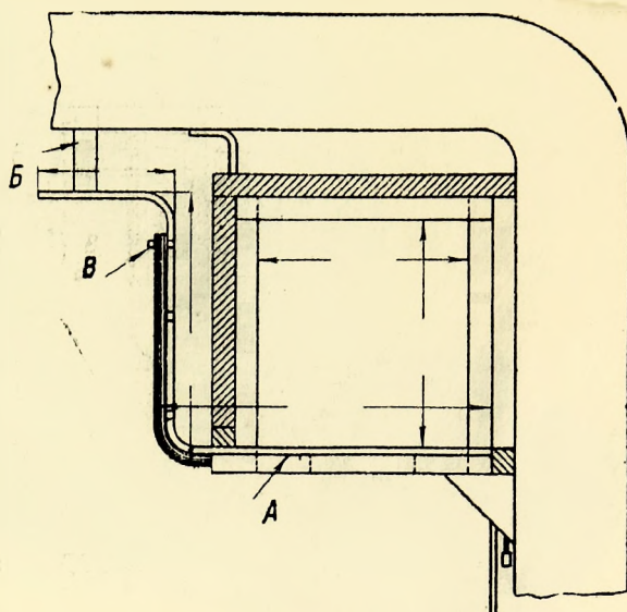
Фиг. 160. Сечение вентиляционного канала в автохолодильнике Сперлинг.
