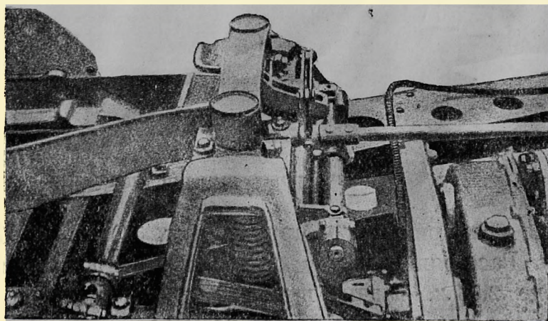
Фиг. 52. Самосцепляющееся тормозное устройство в тягаче Каррьер.
