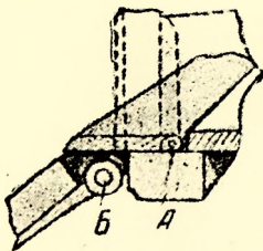
Фиг. 108. Деталь крепления загонных площадок к кузову.
