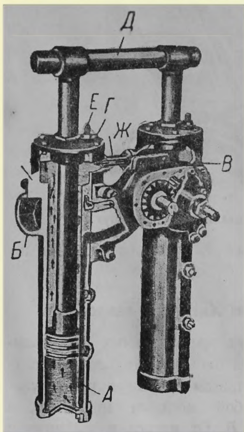
Фиг. 19. Разрез гидравлического под'емного механизма Хилл.
