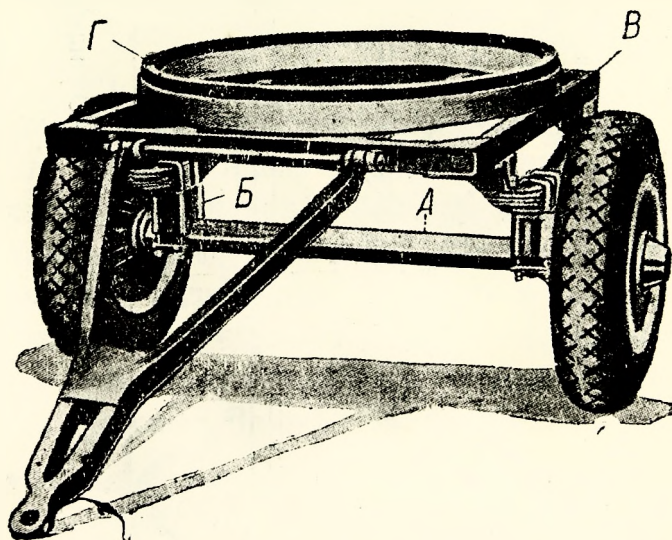
Фиг. 76. Прицепной поворотный скат Дайсон.
