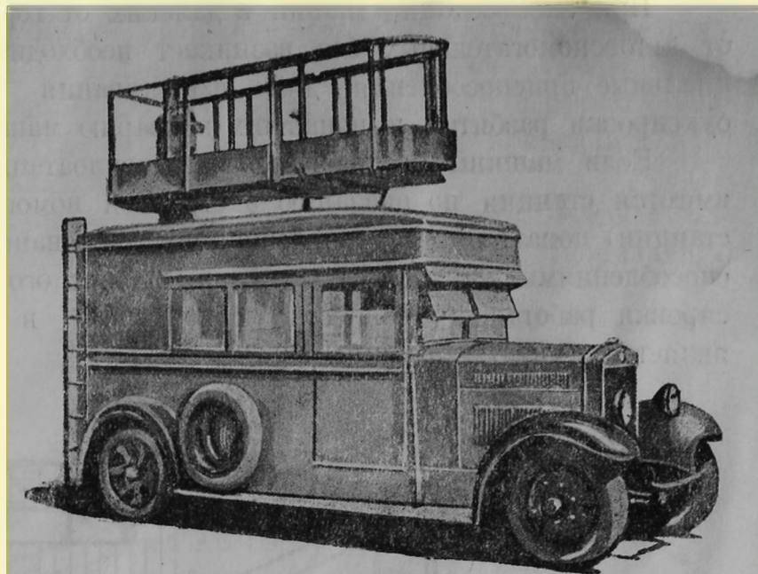
Фиг. 163. Автомобиль Фиат с опущенной телескопической площадкой.
