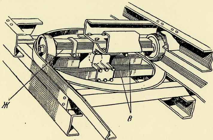
Фиг. 83. Частичный разрез собранной сцепки Бифлекс.
