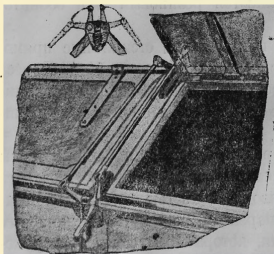
Фиг. 147. Детали действующего от руки устройства для открывания люков в глухих прицепах для перевозки мусора.
