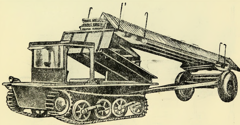
Фиг. 59. Передний вид тягача с полуприцепкой Виккерс.
