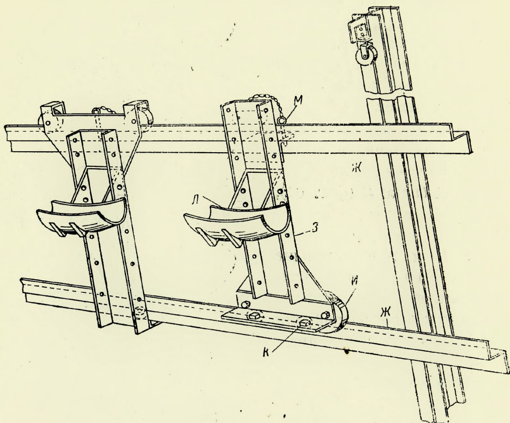
Фиг. 64. Часть рамы полуприцепки Риды с опорными тележками для задних колес автомобилей.
