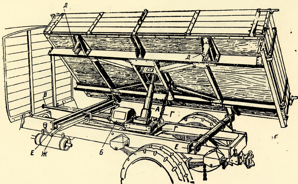
Фиг. 7. Телескопический опрокидывающий механизм Теннер.
