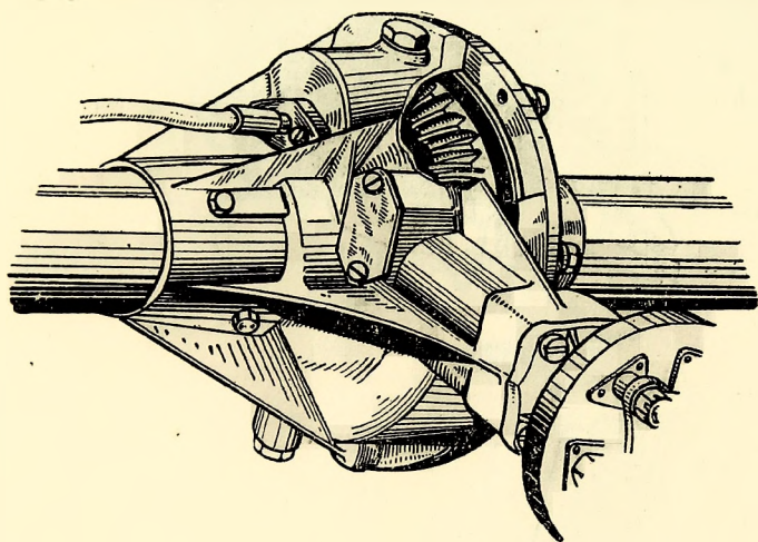
Фиг. 92. Дифференциал втуляторки Ралеих.
