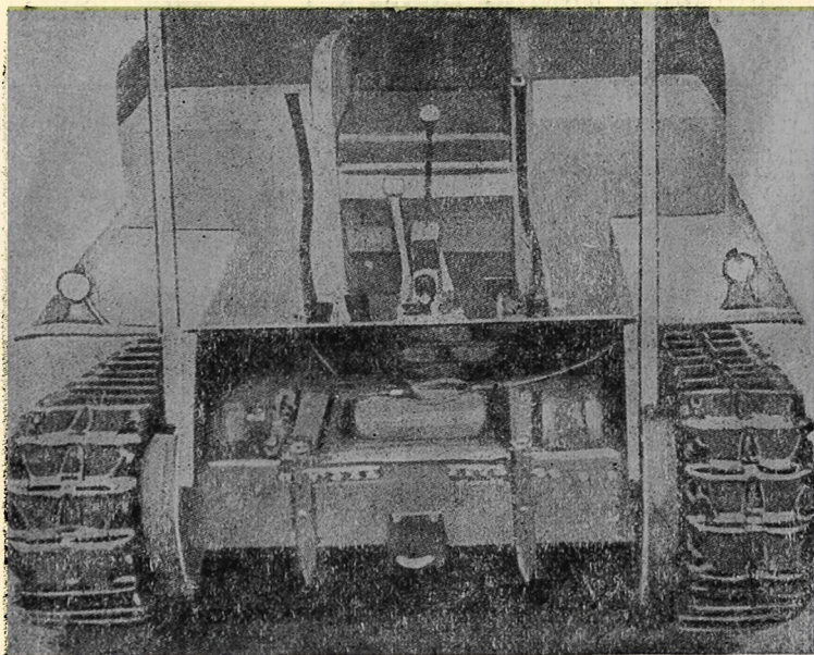
Фиг. 56. Передний вид гусеничного тягача Гаррет-Гарднер.
