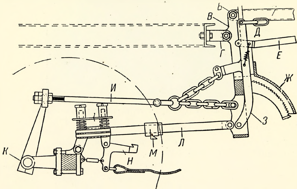
Фиг. 88. Схема устройства автоматических тормозов Прожектайл для прицепок.
