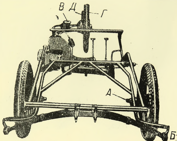
Фиг. 99. Шасси вуатюретки Виктория.
