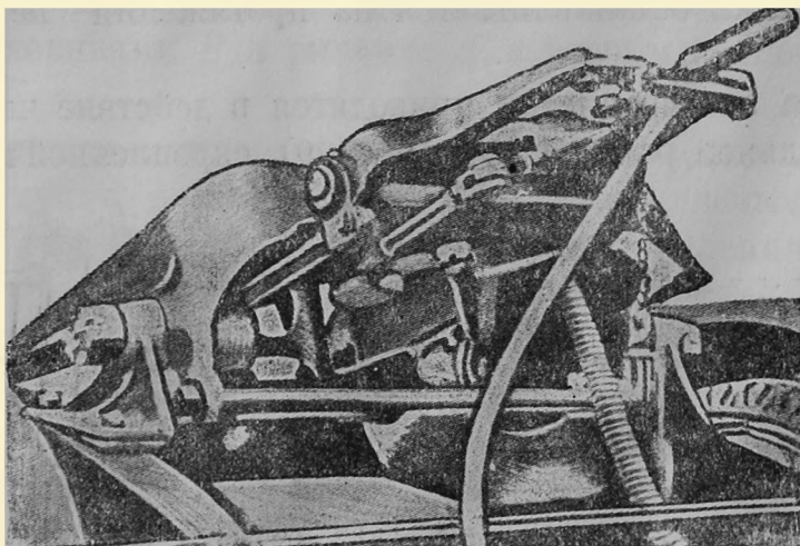
Фиг. 87. Сцепка Брокгауз с тормозным серво-цилиндром.
