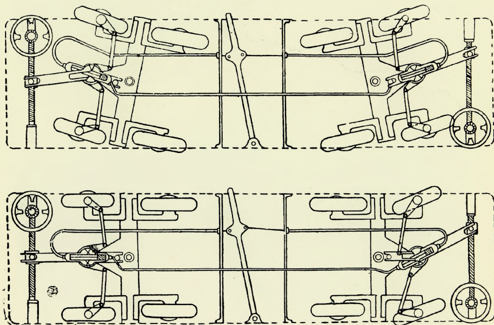
Фиг. 61. Схема поворачивания колес прицепки Джонгофф.
