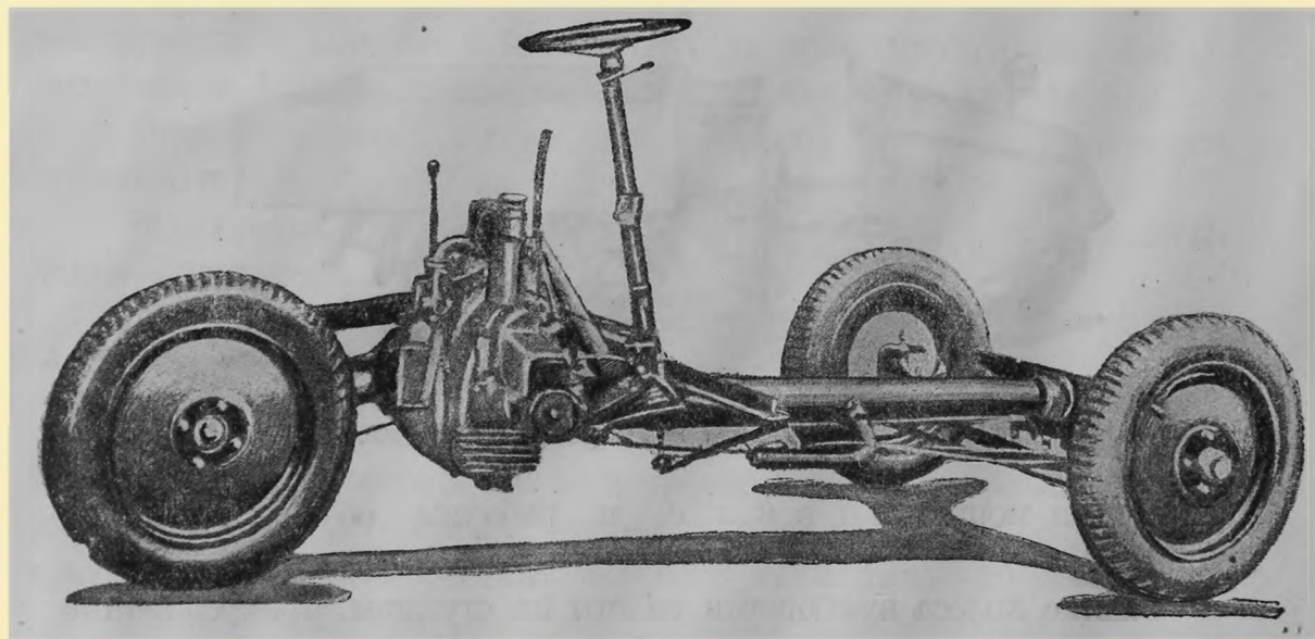
Фиг. 97. Шасси виаютюретки Татра.
