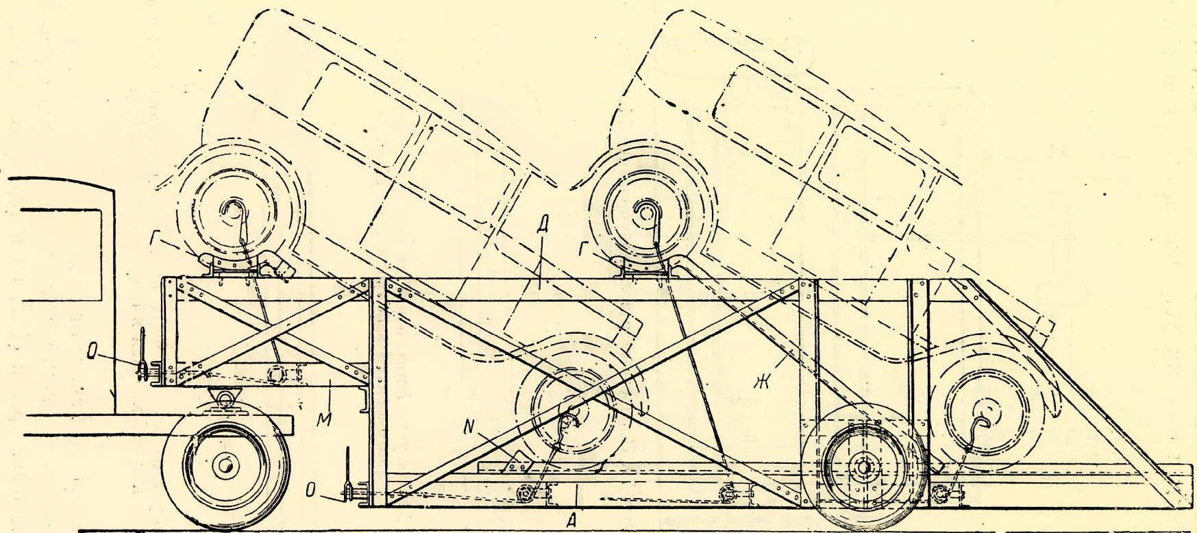
Фиг. 69. Полуприцепка Мак-Гри с погруженными автомобилями.
