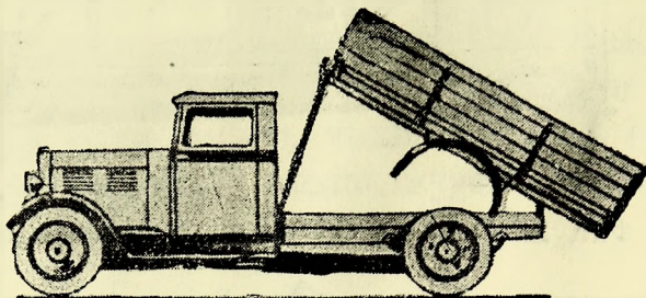
Фиг. 10. Первая система подвешивания кузова к раме автомобиля. Рама отступает от кузова примерно на 20% длины последнего.
