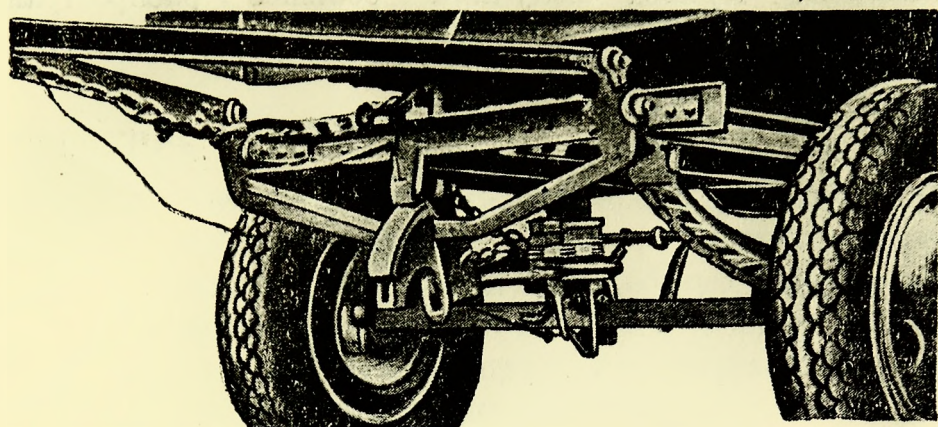
Фиг. 89. Автоматические тормоза Прожектайл для прицепок.
