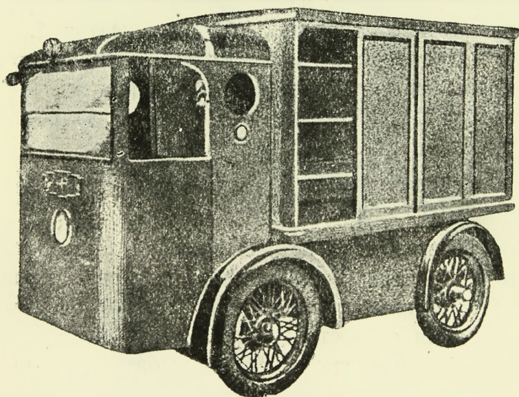
Фиг. 101. Электрическая виаютуретка Моррисон.
