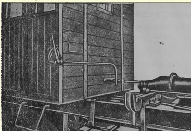
Фиг. 24. Наружное расположение рычага управления самосвалом Вуд.
