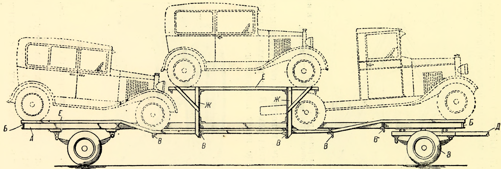
Фиг. 74. Прицепка Эйчильбергера для перевозки автомобилей.
