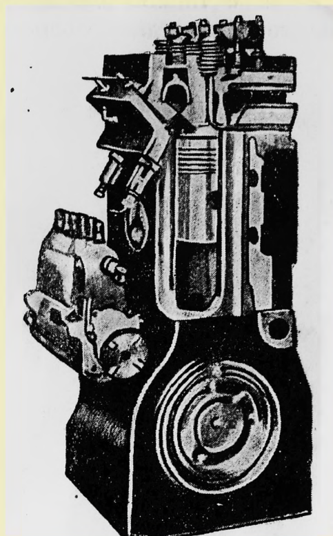
Фиг. 33. Двигатель вездехода Армстронг-Заурер.
