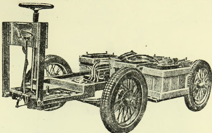
Фиг. 100. Шасси электрической грузовой виаютуретки Моррисон.
