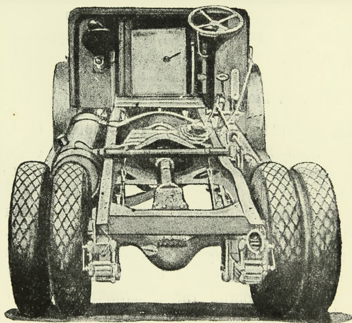
Фиг. 45. Задний вид тягача Гюй.
