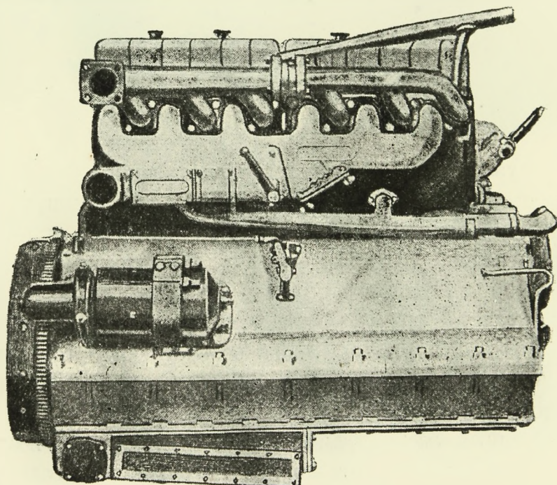
Фиг. 38. Правая сторона дизеля вездехода Кросслей.
