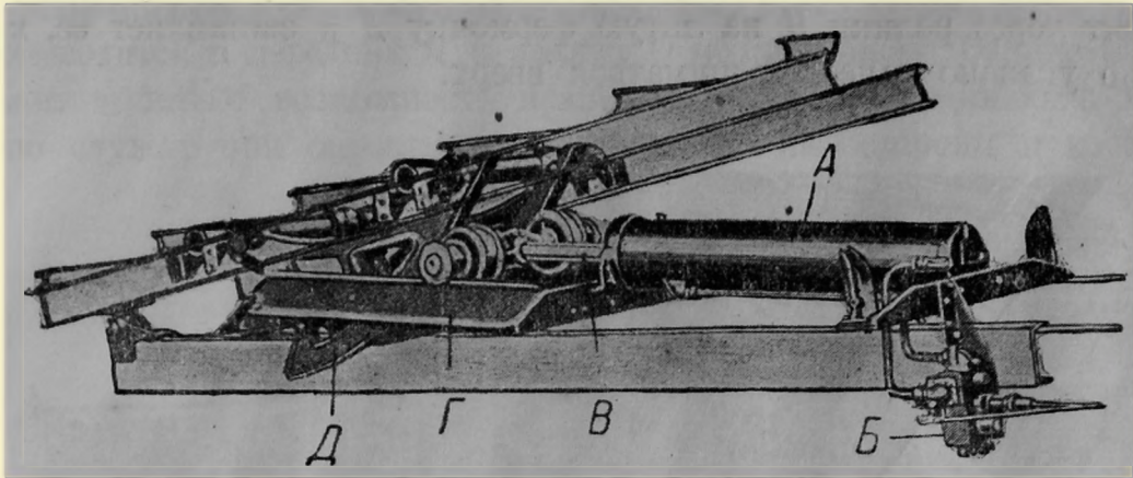
Фиг. 21. Горизонтальный механизм Вуд, опрокидывающий кузов назад.
