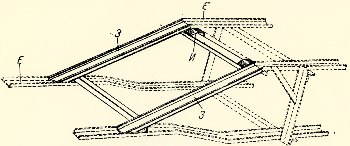
Фиг. 75. Отъемные швеллерные укосины для вкатывания и выкатывания автомобилей в прицепке Эйчильбергера.
