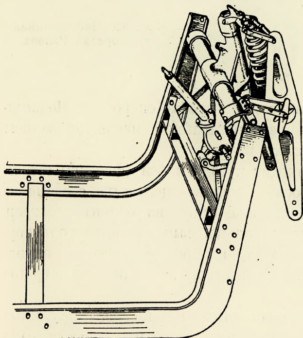
Фиг. 95. Передняя часть рамы с амортизационным устройством в втулочки Ралеих.
