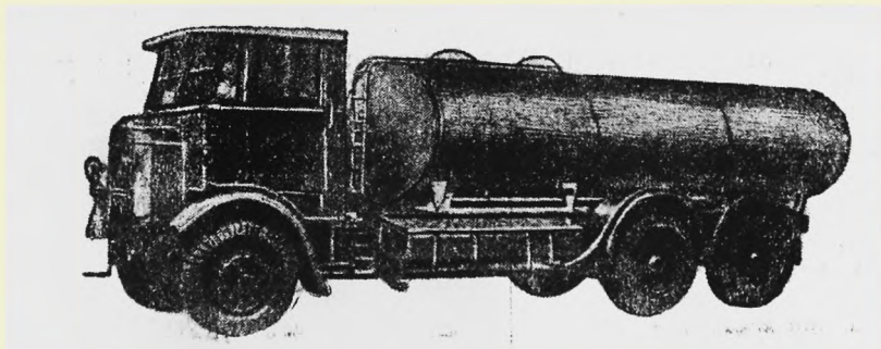
Фиг. 152. Цистерна для молока емкостью в 8500 литров на трехосном шасси Альбион.
