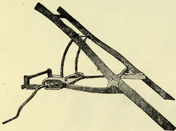
Фиг. 2. Ручной самосвал Брокгауз, приспособленный к 5-тонной прицепке..
