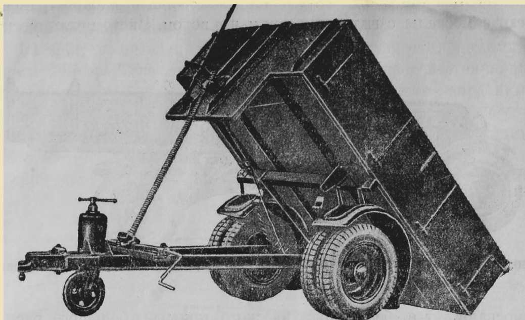
Фиг. 2. Ручной самосвал Брокгауз, приспособленный к 5-тонной прицепке..
