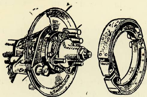
Фиг. 93. Детали устройства тормозов на полуосях втулочки Ралеих.
