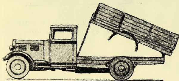
Фиг. 11. Вторая система подвешивания кузова к раме автомобиля. Кузов подвешен почти в задней точке рамы.
