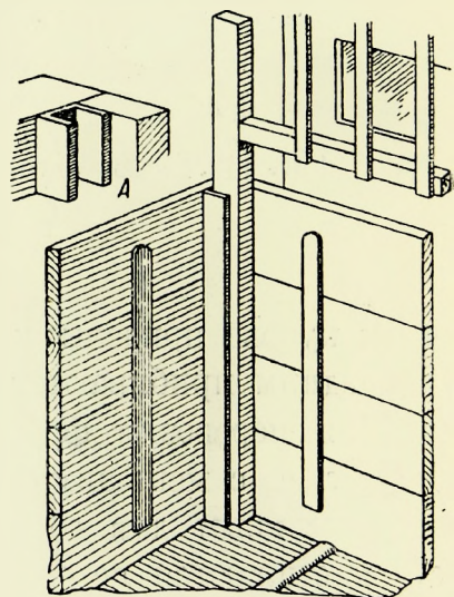
Фиг. 116. Детали крепления съемных боковин в кузове, приспособленном для перевозки овощей и фруктов.
