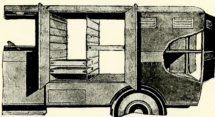
Фиг. 135. Кузов для перевозки хлебных продуктов с боковыми и задними распахивающимися дверцами.
