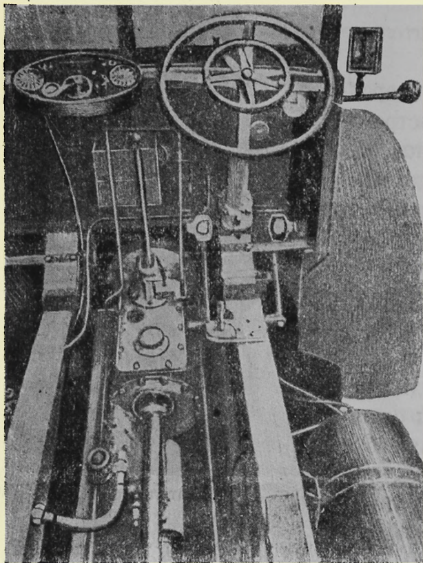
Фиг. 34. Рулевое управление, коробка скоростей и тормозной компрессор вездехода Армстронг-Заурер.
