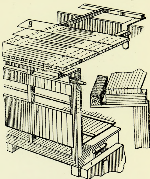
Фиг. 114. Второй способ устройства вспомогательных настилов в кузове, приспособленном для перевозки различных овощей и фруктов.
