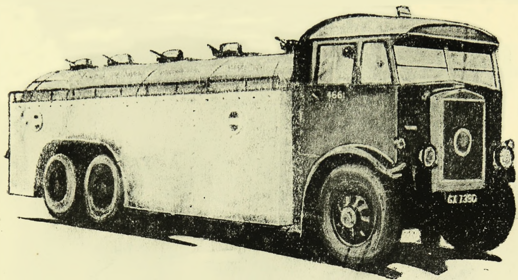
Фиг. 153. Передний вид цистерны Томсон емкостью в 9250 литров на трехосном автомобиле Лейланд.
