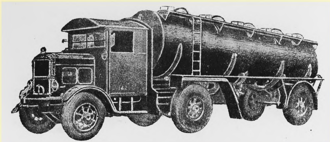
Фиг. 151. Цистерна для бензина емкостью в 9200 литров на полуприцепке с тягачом Скаммель,
