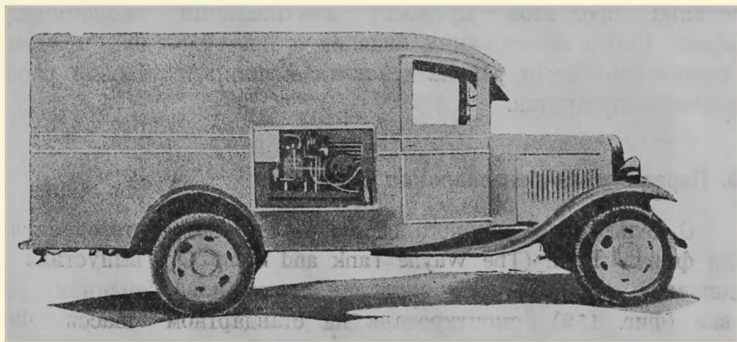
Фиг 159. Автомобиль с рефрижераторной установкой Сперлинг.
