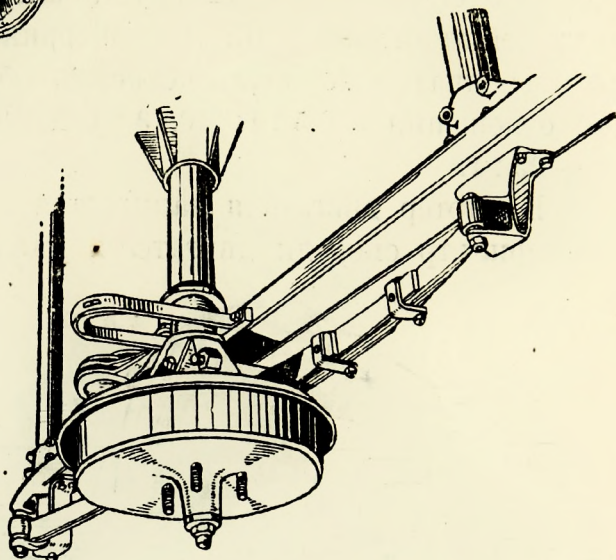
Фиг. 94. Рессоры и задняя полуось втулочки Ралеих.
