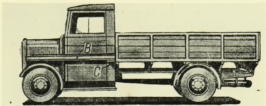
Фиг. 120. Автомобиль со вспомогательным лотком впереди кузова для перевозки длинных предметов.
