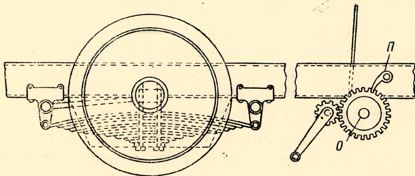
Фиг. 68. Схема устройства подъемного механизма в полуприцепке Рида.
