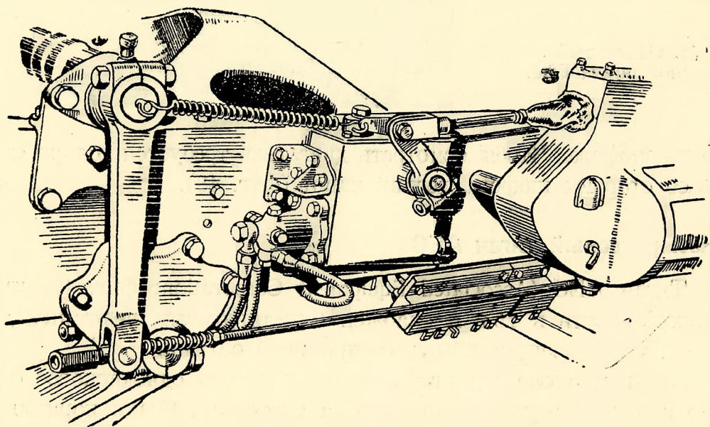
Фиг. 46. Тормозные рычаги и тяги тягача Гюй.
