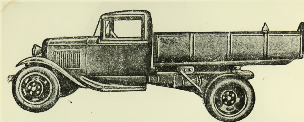
Фиг. 5. Грузовик Форд с ручным самосвалом при горизонтальном положении кузова.
