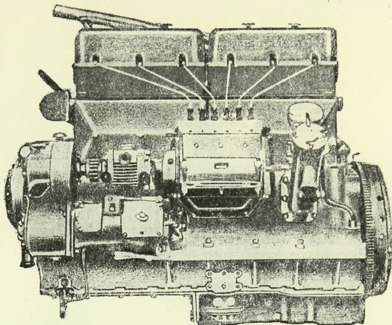
Фиг. 37. Левая сторона дизеля вездехода Кросслей.
