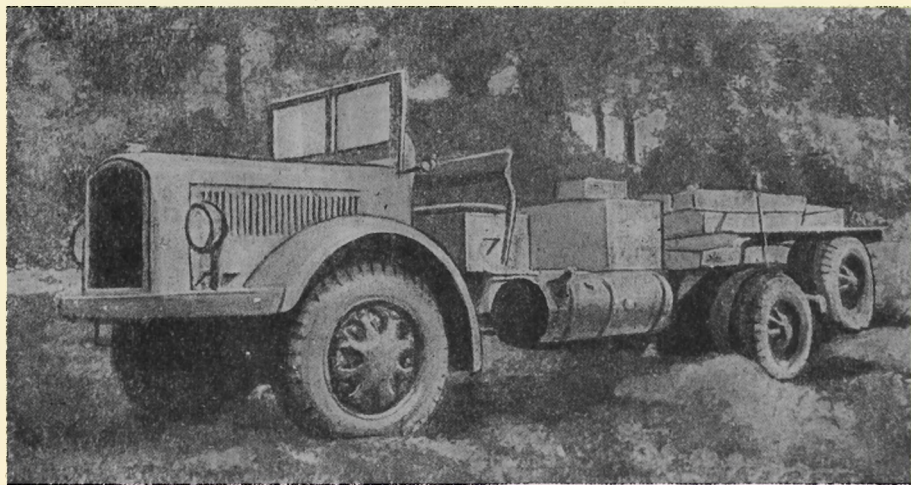
Фиг. 32. Общий вид дизельного вездехода Армстронг-Зауер.
