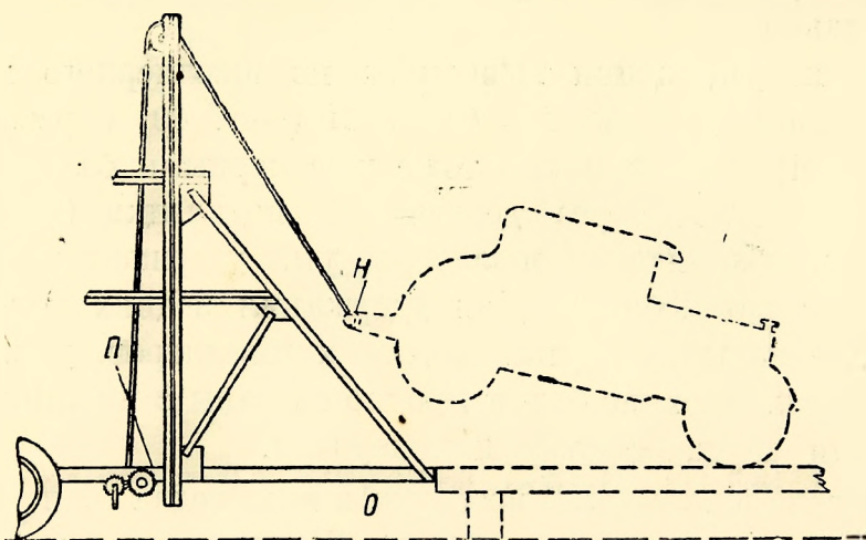
Фиг. 67. Схема закрепления автомобиля в полуприцепке Рида.
