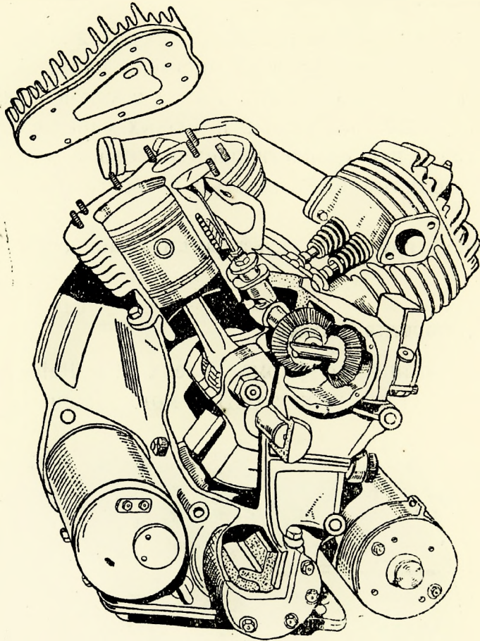
Фиг. 91. Двигатель вуатюретки Раленх.
