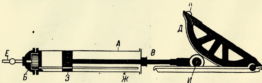
Фиг. 22. Схема устройства механизма Вуд, опрокидывающего кузов назад и на обе стороны.
