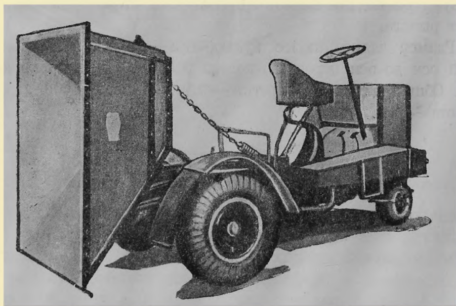
Фиг. 103. Вуатюретка Милларс с опрокинутым кузовом.
