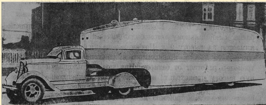
Фиг 161. Полуприцепка с киноустановкой Мак-Колл на тягаче Додж.
