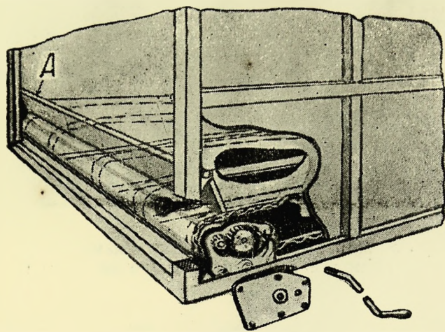
Фиг. 27. Приводное устройство конвейерного самосвала Принсипейлити.
