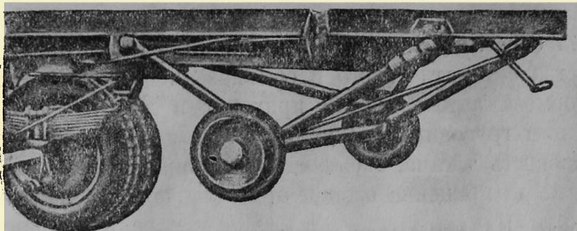
Фиг. 86. Передние откидные колеса полуприцепки Брокгауз.
