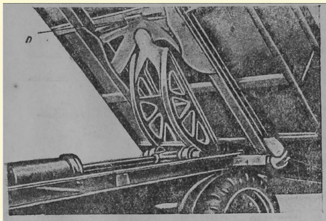
Фиг. 23. Механизм Вуд при опрокидывании кузова назад.
