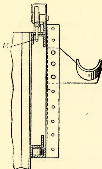
Фиг. 65. Продольное сечение одной из двух передних опорных тележек полуприцепки Рида.
