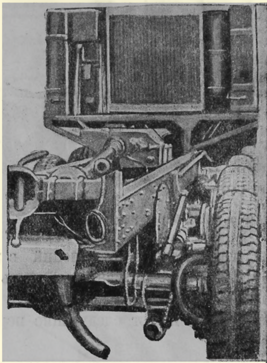
Фиг. 50. Задний вид тягача АЕС.
