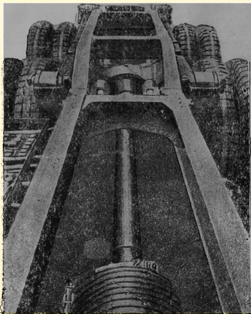
Фиг 36. Карданный вал вездехода Арм-стронг-Заурер.
