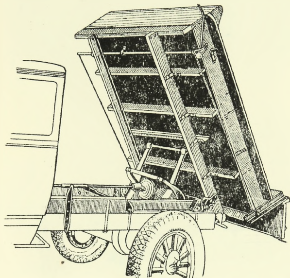
Фиг. 8. Момент опрокидывания кузова гидравлическим механизмом Хилл.
